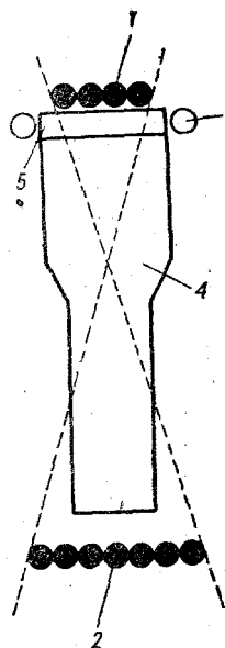
Рис. 6. Схематическое изображение установки для регистрации ядер первичного космического излучения. 1, 2 — счетчики телескопа, выделяющего направление частицы; 3 — боковые счетчики, дающие отметку в случае прихода боковых ливней; 4 — фотоумножитель; 5 — детектор излучения Вавилова — Черенкова. Зачерненные счетчики 1 и 2 включаются в схему двукратных совпадений; кроме того, фиксируется срабатывание более чем одного счетчика в каждой из групп 1 и 2, чтобы исключить случаи прохождения через установку ливней.
