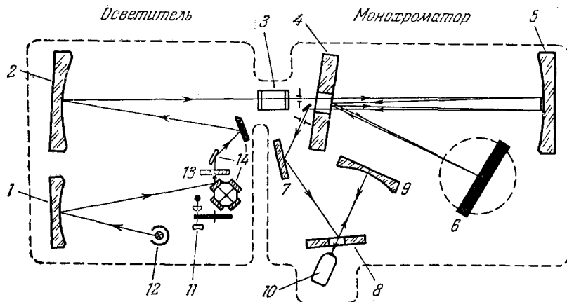
Рис. 18. Оптическая схема спектрометра ДИКС-1 64 : 1, 2, 5, 9 — сферические зеркала; 6, 7, 8 — плоские зеркала; 3 — газовая кювета; 4 — эшелетт; 10 — приемник радиации; 11 — устройство для получения опорного напряжения синхронного детектора; 12 — источник радиации; 13 — кристаллический модулятор; 14 — отражающие фильтры.
