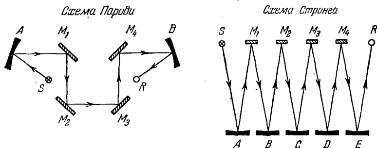
Рис. 4. Метод остаточных лучей 16 ; M_1, M_2, M_3, M_4 — кристаллы, A, B, C, D, E — сферические зеркала, R и S — приемник и источник радиации.
