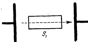
Рис. 3. Устройство для ускорения вращающегося электрически заряженного цилиндра.
