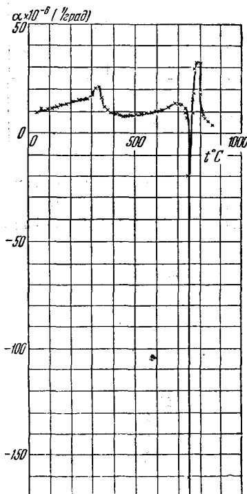
Рис. 11. Зависимость коэффициента линейного расширения поликристаллического образца трехокиси вольфрама от температуры 30 .
