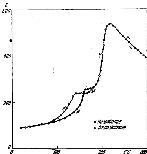
Рис. 9. Зависимость начальной диэлектрической проницаемости поликристаллического образца PbNiO 3 от температуры 27 .
