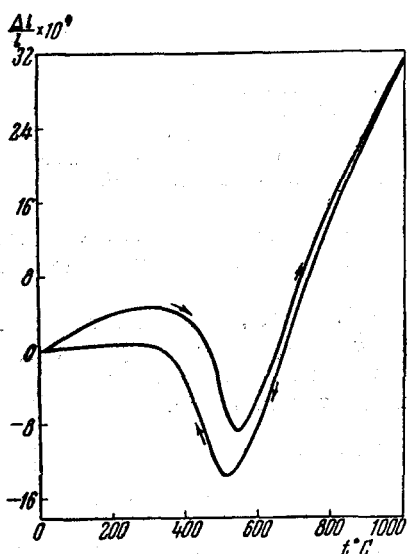
Рис. 14. Зависимость относительного изменения длины поликристаллического образца метаниобата свинца от температуры 42 .
