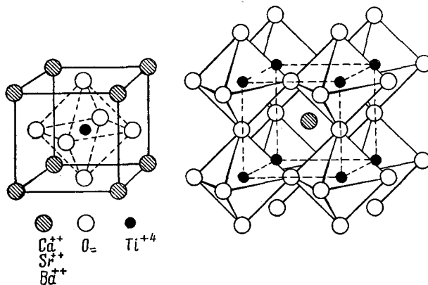
Рис. 1. Расположение ионов в соединениях CaTiO_3 , SrTiO_3 , BaTiO_3 со структурой типа перовскита.
