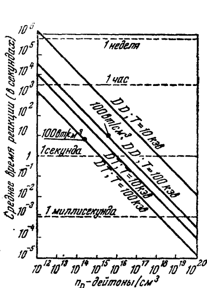
Рис. 4. Зависимость среднего времени реакции от концентрации частиц дейтерия, вычисленная для различных температур.
