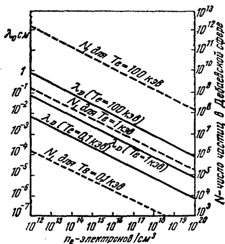
Рис. 8. Зависимость длины волны Дебая и числа частиц внутри дебаевской сферы от концентрации частиц.
