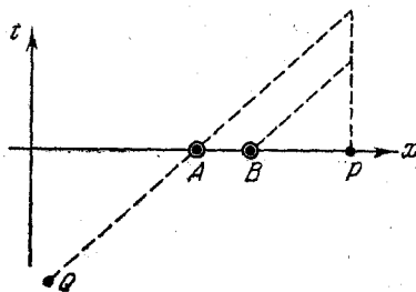
Рис. 2. Распространение сигнала от протяженной частицы. Q — источник волны; A, B — структурные элементы частицы AB ; P — удаленная от AB точка наблюдения.
