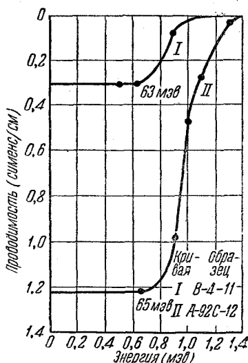
Рис. 11. Проводимость двух образцов германия после бомбардировки электронами в зависимости от энергии электронов (по Клонтцу 119 a).
