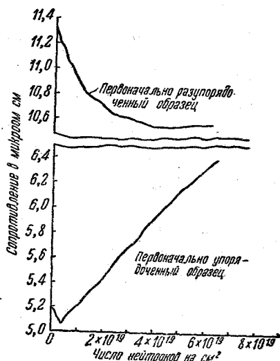
Рис. 2. Изменение сопротивления разупорядоченного и упорядоченного образцов \text{Cu}_2\text{Au} во время нейтронной бомбардировки при 80^\circ\text{C} (Глик, Брукс, Витциг и Джонсон 84 ).
