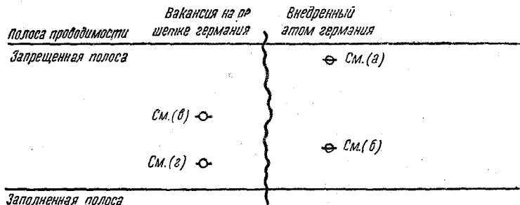
Рис. 10. Диаграмма уровней для вакансий и внедренных атомов в германий; (а) Если уровень занят, атом внедрения нейтрален; (б) если уровень свободен, атом внедрения дважды заряжен; (в) если уровень занят, вблизи вакансии имеется заряд, равный заряду двух электронов; (г) если уровень свободен, вблизи вакансии заряд равен нулю.
