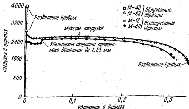
Рис. 7. Кривые удлинения под нагрузкой облученного и необлученного молибдена при комнатной температуре (Брэч, Макхью и Хокенбери 33б ).
