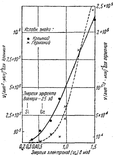
Рис. 12. Наклон \gamma графика « (J_s)^{-2} — время», который должен был быть пропорциональным числу имеющихся дефектов, в зависимости от энергии бомбардирующих электронов (Лоферский и Раппапорт [36]).
