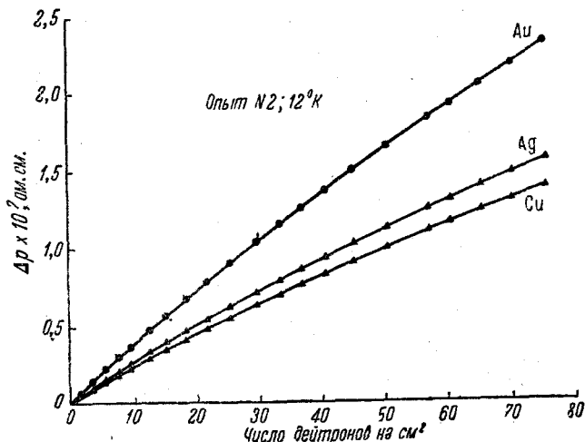
Рис. 1. Увеличение сопротивления меди, серебра и золота во время бомбардировки дейтронами с энергией 12 Мэв при 12^\circ \text{K} (Купер, Кёлер и Маркс 466 ).
