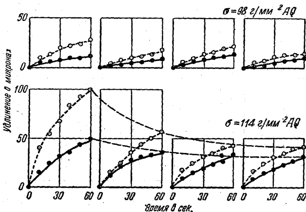
Рис. 5. Кривые текучести кристаллов цинка при облучении альфа-частицами (●—●) и без облучения (○—○). Образцы испытывались без облучения в течение 1 минуты, затем перерыв в течение 3 минут, испытание при облучении, перерыв 3 минуты и т. д. (Шмид и Линтнер 192б ).
