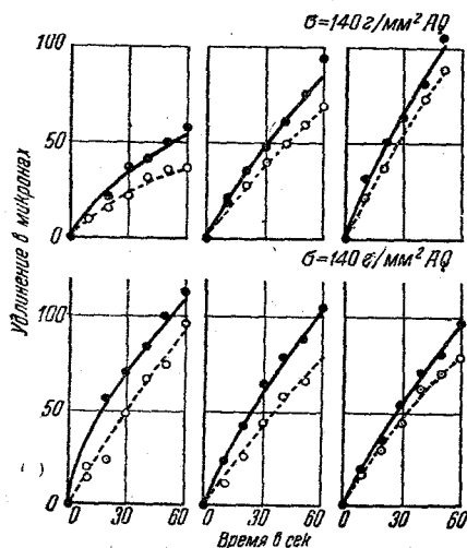
Рис. 6. Кривые текучести кристаллов цинка при облучении нейтронами от радон-бериллиевого источника (●—●) и без облучения (○—○). Метод испытания такой же, как и в опытах, представленных на рис. 5 (Шмид и Линтнер 1926 ).
