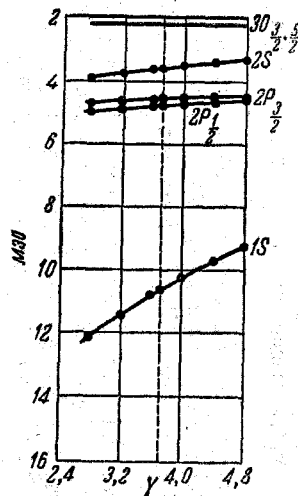
Рис. 6. Зависимость уровней энергии \mu -мезона в поле равномерно заряженного ядра Rb от радиуса ядра. Ординаты — энергия в Мэв. Абсциссы — радиус в единицах \pi = 1,87 \cdot 10^{-13} см.
