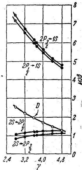
Рис. 7. Зависимость энергий переходов 2P-1S , 2P-2S и дублетного расщепления от радиуса равномерно заряженного ядра. Ординаты — энергия в Мэв. Абсциссы — радиус в единицах \lambda = 1,87 \cdot 10^{-13} см, D — дублетное расщепление 2P_{3/2} - 2P_{1/2} , увеличенное в 10 раз.
