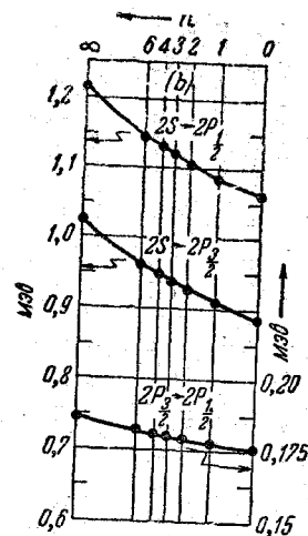
Рис. 8. Зависимость энергий переходов 2S-2P_{1/2} , 2S-2P_{3/2} и дублетного расщепления 2P_{3/2}-2P_{1/2} от формы плотности заряда f(x) при фиксированной энергии перехода 2P_{3/2}-1S 6,00 Мэв. Ординаты — энергия в Мэв. Левая шкала — для переходов 2S-1P . Правая шкала — для дублетного расщепления. Абсциссы — параметр n . n = \infty соответствует прямоугольному распределению, n = 1 — экспоненциальному.
