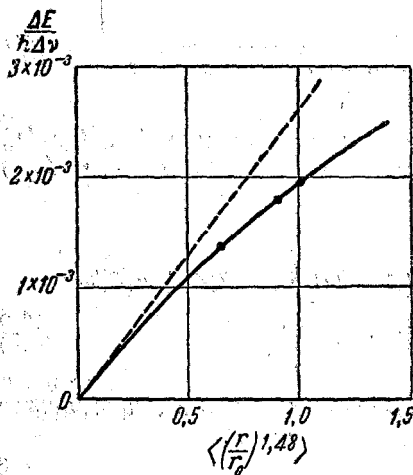
Рис. 5. \frac{\Delta E}{h\Delta\nu} как функция от \langle r^{1,48} \rangle при Z = 92 . Абсциссы — \left\langle \left( \frac{r}{r_0} \right)^{1,48} \right\rangle , где r_0 = 1,5 \cdot 10^{-13} (238)^{1/3} см.
