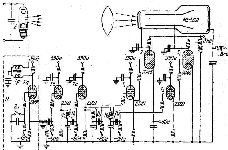
Рис. 5. Схема для получения однократных снимков с выдержкой от 3 \cdot 10^{-8} до 2 \cdot 10^{-6} сек с преобразователем МЕ-1201.
