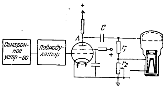
Рис. 1. Схема импульсного включения электроннооптического преобразователя типа AEG.
