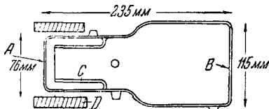
Рис. 18. Электроннооптический преобразователь типа МЕ-1200, предназначенный для получения развёртки изображения с помощью магнитного отклонения.
