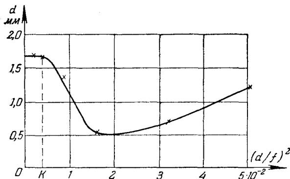
Рис. 15. Зависимость диаметра изображения канала искрового разряда на экране преобразователя от уровня освещенности на фотокатоде.
