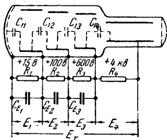
Рис. 2. Делитель напряжения для импульсного включения преобразователя типа 1P25.
