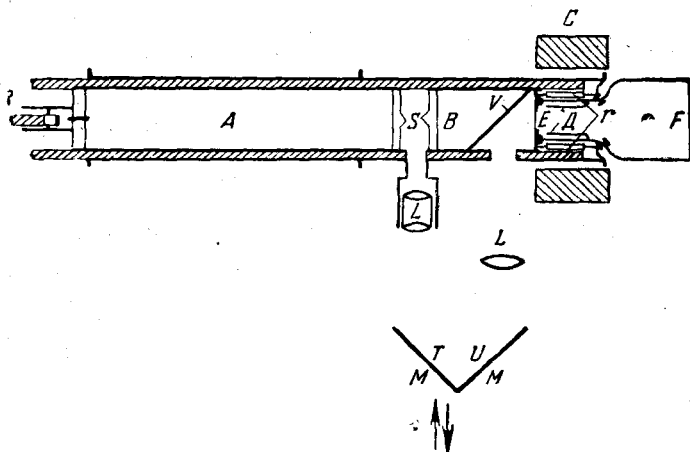
Рис. 9. Схема установки для изучения стримерного разряда.
