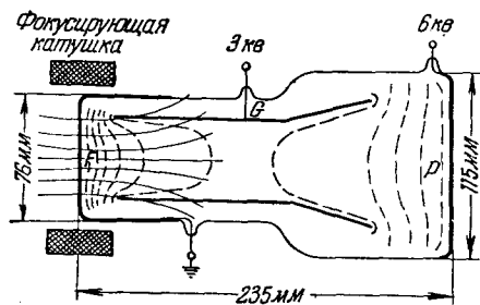
Рис. 3. Трёхэлектродный электроннооптический преобразователь типа МЕ-1201 с комбинированной электростатической и магнитной фокусировкой.
