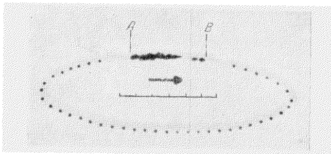
Рис. 23. Эллиптическая развёртка свечения, возникающего при разряде вибратора Лебедева, длиной 12 мм, в азоте при давлении 30 атм. Одно деление шкалы соответствует 1 \cdot 10^{-10} сек. Полная длительность свечения искры 4,5 \cdot 10^{-10} сек.
