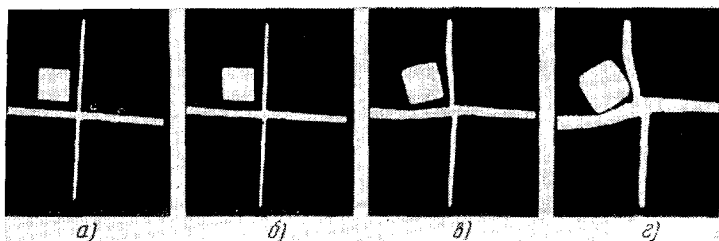
Рис. 13. Искажения изображения, возникающие на экране преобразователя ME-1201 при сильном местном освещении фотокатода. (а) — изображение мира, проектируемой на фотокатод, (б), (в), (г) — изображение мира на экране преобразователя при импульсном его включении и различных уровнях освещённости фотокатода. Освещённость в (в) и (г) соответственно в 2 и 4 раза больше, чем в (б).
