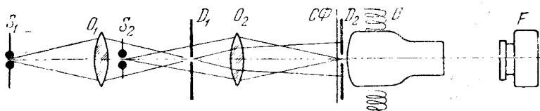
Рис. 21. Схема оптической установки для фотографирования с экрана электроннооптического преобразователя развёртки ударной волны и свечения, возникающих при искровом разряде.
