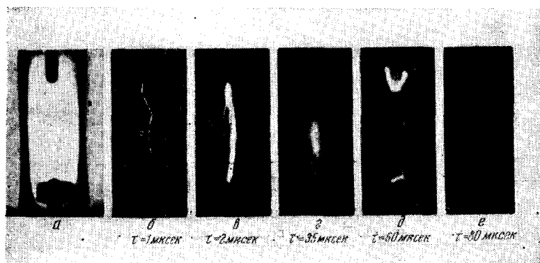
Рис. 6. Различные стадии свечения разряда в импульсной лампе LSD2, снятые через электроннооптический преобразователь ME-1201 с выдержкой 0,1 \mu\text{сек} . а — расположение электродов в лампе; б, в, г, д, е — свечение лампы в различные моменты времени от начала разряда.
