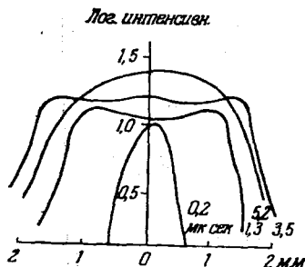
Рис. 8. Распределение интенсивности излучения в канале искрового разряда в водороде. Давление p = 760 мм; I = 1500 а, выдержка t = 0,5 мксек.
