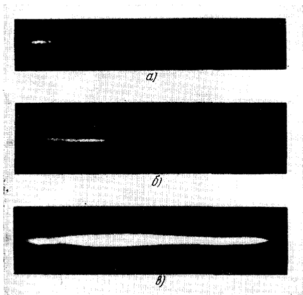
Рис. 10. Рост стримера искрового разряда. Электронно-оптический преобразователь открывается на промежуток времени порядка 4,5 \cdot 10^{-9} \text{ сек} . Относительная задержка во времени (а)—0; (б)— 1,3 \cdot 10^{-9} \text{ сек} ; (в)— 3,4 \cdot 10^{-9} \text{ сек} .
