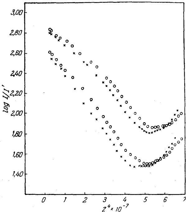
Рис. 5. Кривые обращения при разном содержании озона (обсерватория на горе Абу, Индия). 5.2.1952, x = 0,188 \text{ см} } (верхние кривые 3112 Å/3323 Å). 7.2.1952, x = 0,209 \text{ см} } (нижние кривые 3075 Å/3278 Å).
