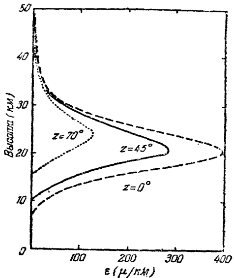
Рис. 37. Вертикальное распределение озона при разном зенитном расстоянии Солнца.
