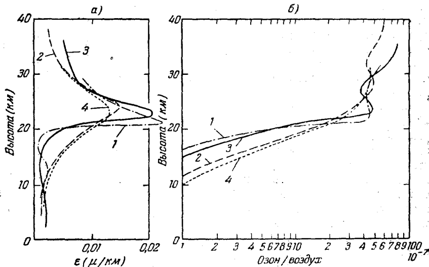
Рис. 56. Вертикальное распределение озона осенью над Вейсенау: 1 — 8.9.1953; 2 — 28.9.1953; 3 — 23.10.1953; 4 — 28.10.1953 (по Петцольду).
