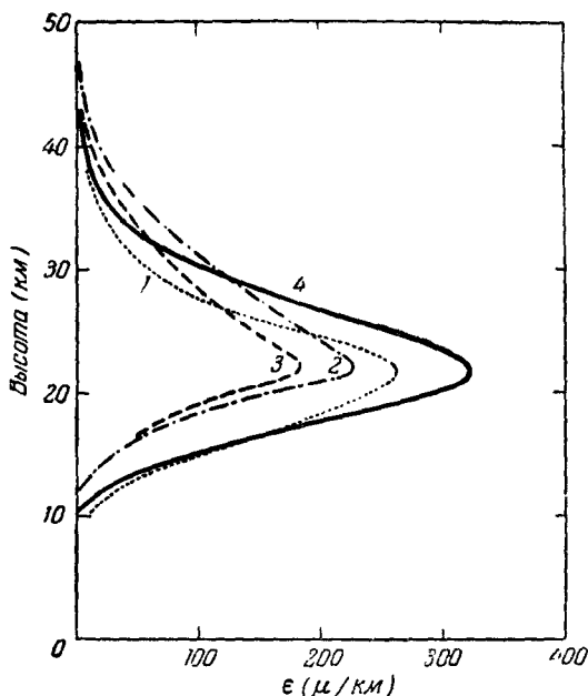
Рис. 35. Вертикальное распределение равновесных концентраций озона, вычисленное по формуле (5.5) при разных предположениях о внеатмосферной интенсивности солнечного излучения (табл. IV) и о зависимости кислородного поглощения от давления (Петцольд).
