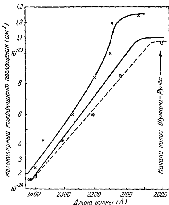
Рис. 30. Коэффициент поглощения кислорода в континууме Херцберга: \circ — по данным А. Васси 40 ; \times — по данным Бюиссона 49 ; — — — кривая, принятая Николе и Манжем 43 .
