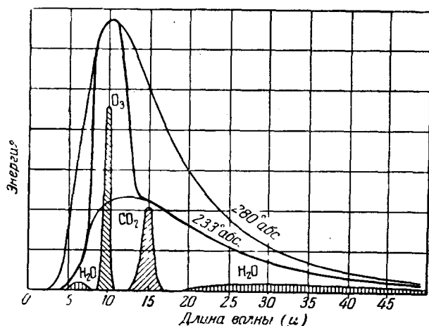
Рис. 62. Примерное распределение энергии в спектре обратного излучения на уровне нижних слоев стратосферы.
