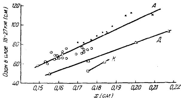
Рис. 57. Количество озона в слое 18—27 км в зависимости от общего содержания озона в атмосфере x (обсерватории Индии) АХ — Абу (февраль — март); АО — Абу (остальные месяцы); ДΔ — Дели; К□ — Кодайканал.
