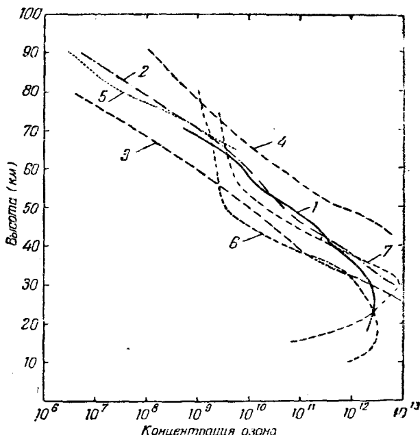
Рис. 39. Сопоставление концентраций озона в верхней части озонного слоя, полученных путём ракетных измерений (кривая 1) и путём расчётов на основе теории фотохимического равновесия; 2 — Джонсон и др. 42 ; 3 — Вульф и Деминг (A); 4 — Вульф и Деминг (D); 5 — Бейтс и Николе; 6 — Дютш; 7 — Крейг.
