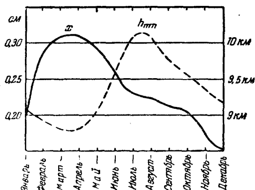
Рис. 44. Средний годовой ход количества озона x и высоты тропосферы h_{mn} над Тромсё (Юхансен).
