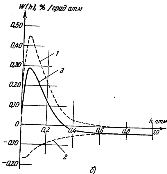
Рис. 1. Плотность температурного коэффициента. а — на уровне моря, б — на глубине 70 м водного эквивалента. Кривая 1 — W_{\pi}(h) ; кривая 2 — W_{\mu}(h) ; кривая 3 — W(h) = W_{\pi}(h) + W_{\mu}(h) .
