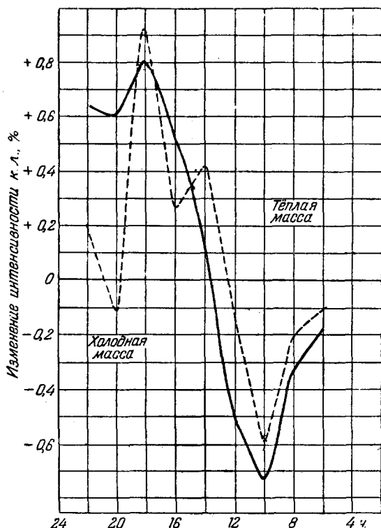
Рис. 6. Прохождение холодного фронта (Якутск, 16 апреля 1951 г.). Сплошная кривая—измерения, пунктир—рассчитанный метеорологический эффект.
