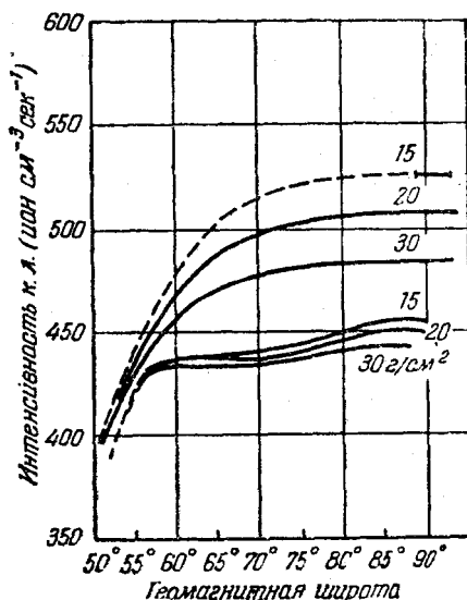
Рис. 15. Изменение широтного эффекта общей ионизирующей компоненты на больших высотах в атмосфере на уровнях с давлением 15, 20 и 30 г/см 2 от лета 1951 г. (нижние три кривые) к лету 1954 г. (верхние три кривые).
