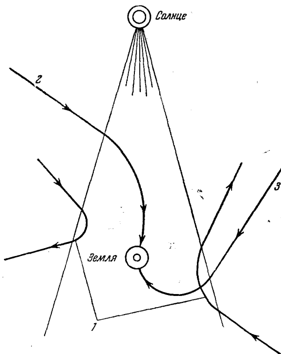
Рис. 13. Эффекты космических лучей во время попадания корпускулярных потоков на Землю (схема). 1 — частицы сравнительно небольшой энергии рассеиваются; их интенсивность на Земле уменьшается; 2 — частицы высоких энергий ускоряющиеся (изменение сказывается на Земле в утренние часы); 3 — частицы высоких энергий замедляющиеся (изменение сказывается на Земле в ночные и вечерние часы).
