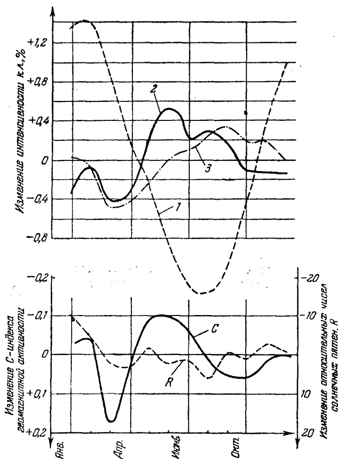
Рис. 9. Годовые вариации космических лучей и магнитная активность. 1 — измерения (Челтенхэм); 2 — метеорологический эффект исключён (Челтенхэм); 3 — измерения (Гуанкайо); C — индекс магнитной активности (левая шкала); R — относительные числа солнечных пятен, числа Вольфа (правая шкала).
