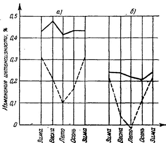
Рис. 4. Зависимость суточных вариаций жёсткой компоненты космических лучей на уровне моря от времени года (Москва): а) разность интенсивностей 14 ч.—2 ч.; б) разность интенсивностей 17 ч.—5 ч. Пунктир—измерения, сплошная кривая — метеорологический эффект исключён.
