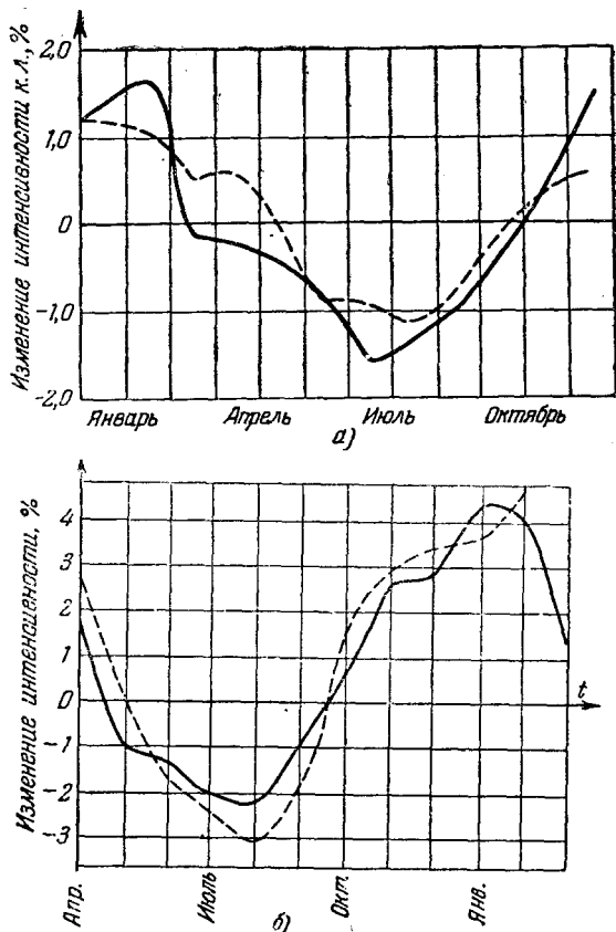
Рис. 2. Сезонные вариации жёсткой компоненты космических лучей на уровне моря: а — в Челтенхэме («одномезонная схема»), б — в Якутск («двухмезонная схема»). Сплошная кривая — эксперимент, пунктир — вклад метеорологического эффекта.
