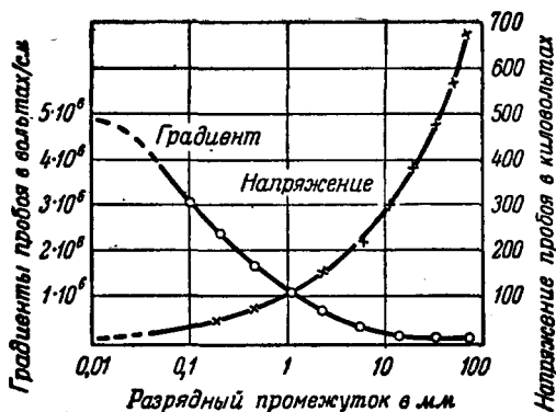
Рис. 1. Пробивные напряжения (крестики) и напряжённости поля (кружки) при пробое в высоком вакууме между стальным шаром диаметром 25,4 мм (анод) и плоским стальным диском диаметром 50,8 мм 6 .
