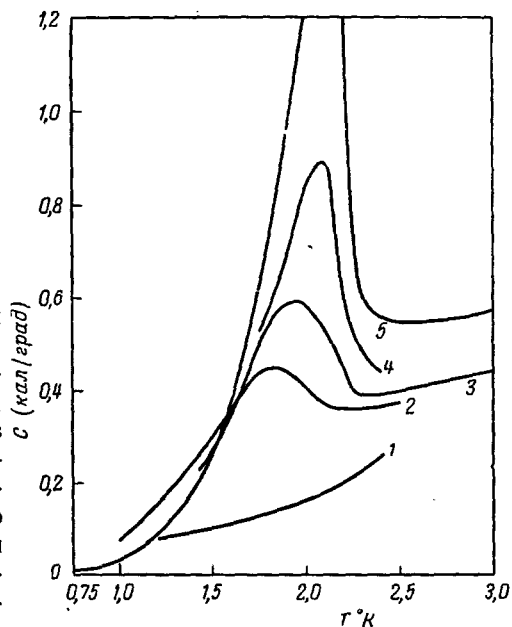
Рис. 32. Теплоёмкость адсорбированного гелия (в кал/град.г) по данным Фредериксе 49a . Кривая 1—3—4 слоя, кривая 2—5—6 слоёв, кривая 3—7—9 слоёв, кривая 4—9—12 слоёв, кривая 5— для жидкого гелия в сосуде. Указанные числа слоёв даны Фредериксе. Относительно новой интерпретации см. раздел 6.3.
