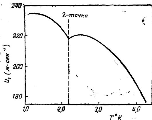
Рис. 48. Скорость первого звука u_1 (м/сек) в жидком гелии по измерениям Аткинса и Чейза А. 51b .
