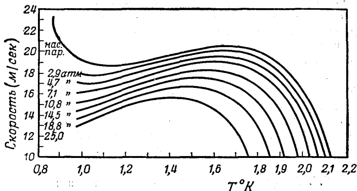
Рис. 52. Скорость второго звука как функция температуры и давления по Мауреру и Херлину М. 51с . Экспериментальные точки общей численностью около 250, хорошо ложащиеся на кривые, не изображены. Максимальное отклонение точек от кривой составляет \pm 1\% . Давления на кривых указаны в атмосферах.
