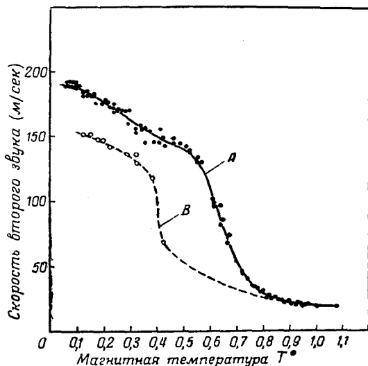
Рис. 51. Скорость второго звука как функция температуры при низких температурах (по де Клерку, Хадсону и Пелламу К. 53а ). Кривая A и соответствующие ей точки — данные де Клерка и др. Пунктирная кривая B и точки на ней — данные Аткинса и Осборна А. 50с .
