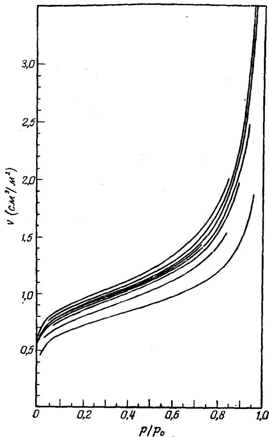
Рис. 36. Изотермы адсорбции гелия на порошке крокуса. Зависимость адсорбированного объёма (в куб. см гелия при нормальных температуре и давлении на 1 \text{ м}^2 адсорбирующей поверхности) от степени насыщения p/p_0 при различных температурах: 4,21^\circ \text{ К} (нижняя кривая), 3,02^\circ \text{ К} , 2,42^\circ \text{ К} , 2,25^\circ \text{ К} , 2,14^\circ \text{ К} , 2,01^\circ \text{ К} , 1,80^\circ \text{ К} и 1,59^\circ \text{ К} (верхняя кривая). Данные Штраусса (см. Лонг и Мейер L. 53a ).
