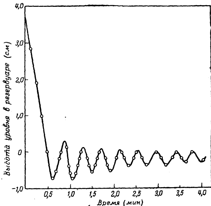
Рис. 35. График, показывающий колебательный характер сверхтекучего вытекания гелия из резервуара при разности уровней, близкой к нулю. Аллен и Майзнер А. 39а.
