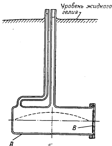
Рис. 53. Схема тепловой трубки Пито-Пеллама Р-50б. Пунктирная кривая внутри горизонтального сосуда А представляет распределение плотности теплового потока (В — плоский электрический нагреватель) при резонансе. Обусловленная этим разность уровней в вертикальных трубках, так же как и подъём вследствие капиллярных сил, здесь преувеличены.
