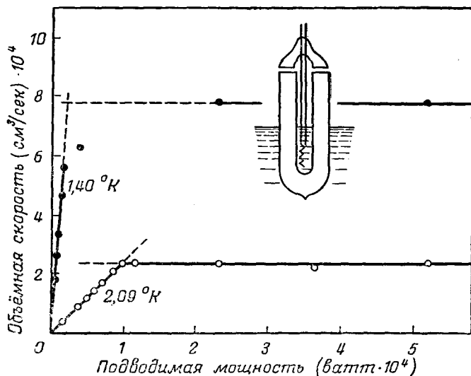
Рис. 47. Прибор и результаты измерений Чандрасекара и Мендельсона 51 , зависимости объёмной скорости перетекания гелия II по плёнке в резервуар от мощности, выделяемой в резервуаре.
