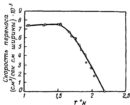
Рис. 39. Зависимость скорости переноса по плёнке на стеклянной поверхности (в \text{см}^3/\text{сек см ширины} ) от температуры (Доунт и Мендельсон D. 39b).
