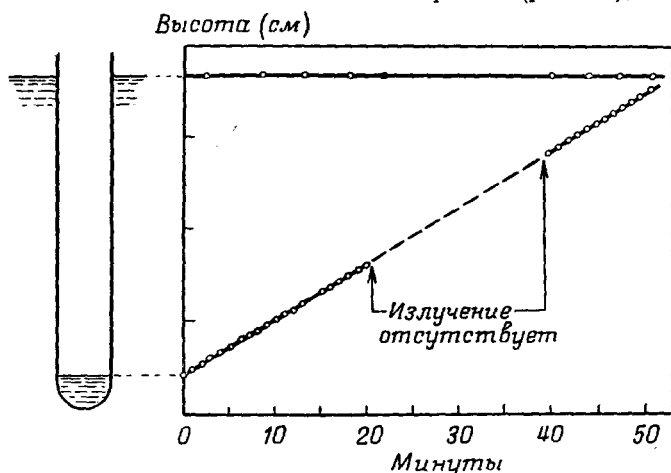
Рис. 42. Типичный результат опытов Бауэрс и Мендельсона В. 50е с прибором, изображённым на рис. 41. На кривой отложена зависимость от времени высоты уровня гелия в пробирке при её наполнении.
