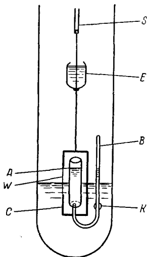
Рис. 46. Прибор Джексона и Хэншоу 1.50 для одновременного измерения скорости переноса и толщины плёнки. A — стальная пробирка со стеклянной трубкой B , присоединённой к ней при помощи спая ковар-стекло K , C — медный экран с окошком W для наблюдения, E — тепловой экран с жидким гелием, S — подвес.
