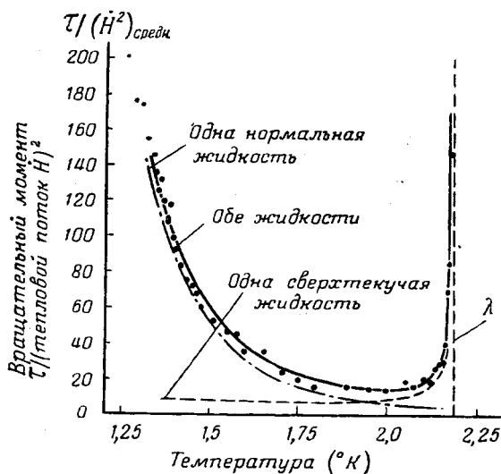
Рис. 55. Отношение \tau/(H^2)_{\text{среди}} как функция температуры T . Кривые соответствуют теоретическим ожиданиям; кружки — наблюдаемые значения.
