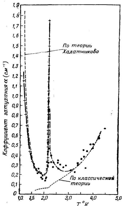
Рис. 49. Коэффициент затухания ультразвука как функция температуры по измерениям Пеллама и Сквайра Р. 47 . В области от 1,6 до 1,2^\circ \text{K} кривая проведена по данным недавней работы Аткинса и Чейза (см. А. 52а). Пунктирная кривая выше 1,6^\circ \text{K} изображает теоретическую кривую для \alpha , вычисленную Пелламом и Сквайром Р. 47 классическим методом. Пунктирная кривая ниже 1,6^\circ \text{K} представляет коэффициент \alpha по вычислениям Халатникова, полученный совмещением его результатов с экспериментальными значениями при высокой температуре по измерениям Аткинса А. 52а . ● — измерения Пеллама и Сквайра Р. 47 , + — измерения Аткинса и Чейза (см. А. 52а).
