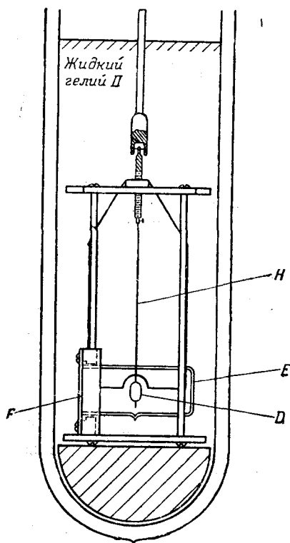
Рис. 54. Схема прибора, использованного Пелламом и сотрудниками P. 52b для экспериментов с диском Рэля в жидком гелии II (см. текст).
