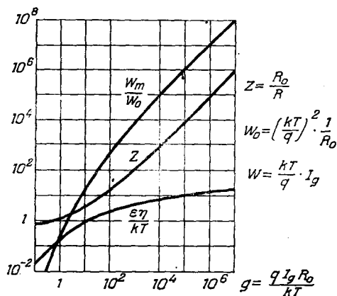
Рис. 3. Зависимость относительной проводимости нагрузки Z , приведённой максимальной мощности \frac{W_m}{W_0} и приведённой предельной эффективности \frac{\varepsilon\eta}{kT} от приведённого тока g .
