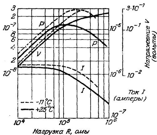
Рис. 6. Преобразование энергии \beta -частиц Si кремниевым э.-д. переходом.
