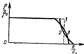
Рис 18. Средняя плотность заряда для деформированных ядер.
