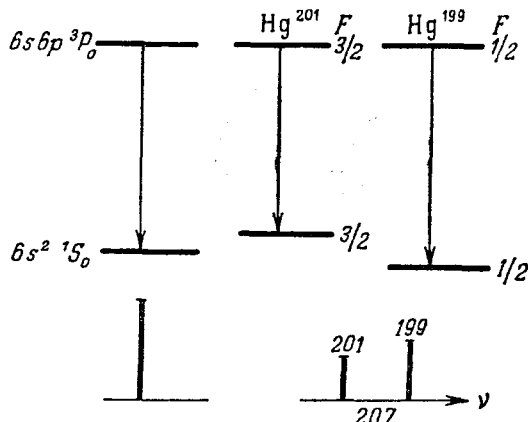
Рис. 9. Схема переходов и структура линии Hg I 2655,8 Å.
