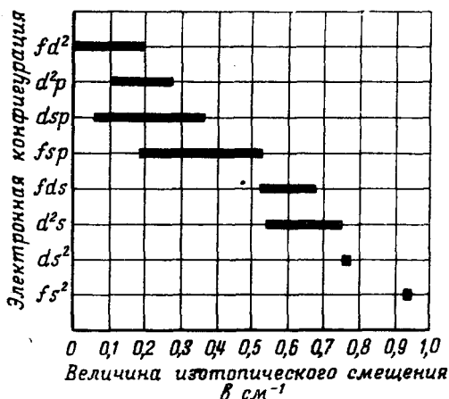
Рис. 13. Изотопическое смещение в термах различных электронных конфигураций Th.
