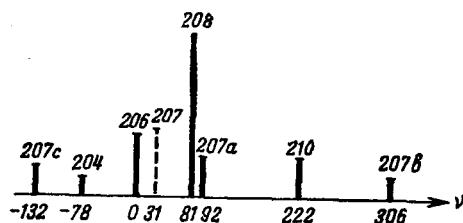
Рис. 11. Изотопическая и сверхтонкая структура линии Pb I 4057,8 Å (пунктирной линией отмечен центр тяжести сверхтонкой структуры изотопа Pb 207 ).
