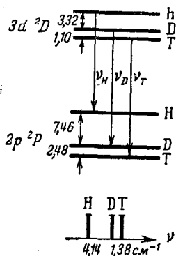
Рис. 1. Схема переходов и изотопическая структура для линии H_\alpha .
