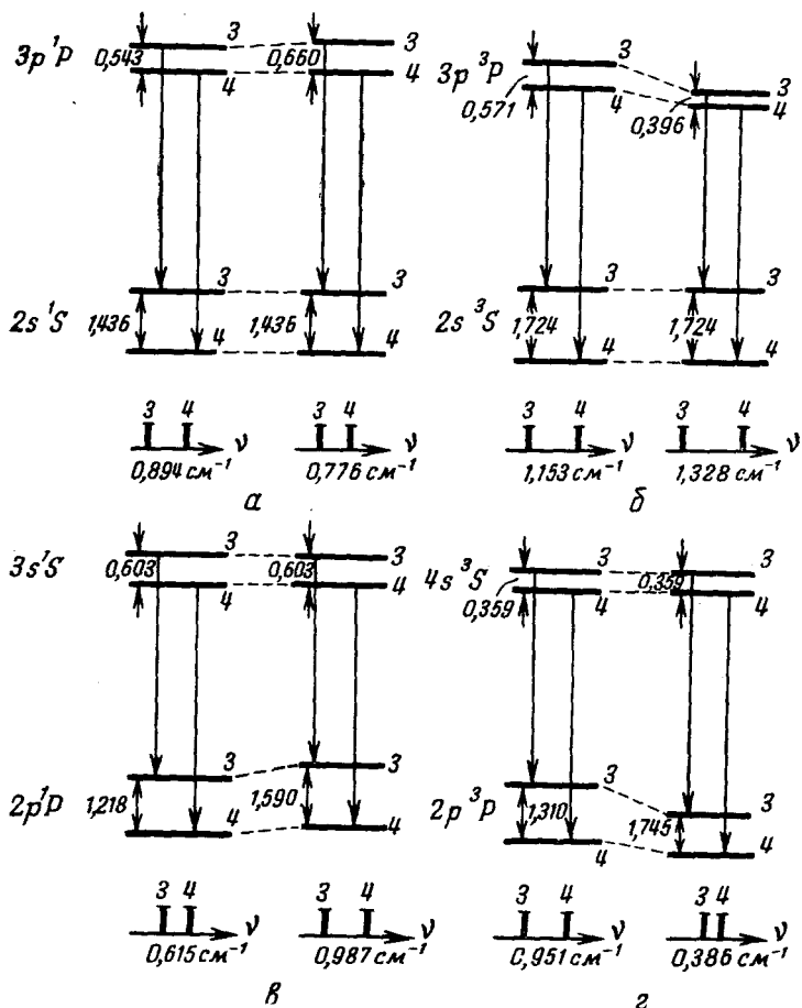
Рис. 3. Схема переходов и изотопическая структура линий гелия:
