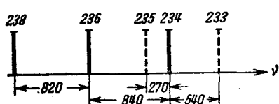
Рис. 14. Изотопическая структура линии U II 4244,4 Å.
