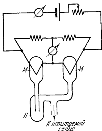
Рис. 2. Схема дифференциального течеискателя.
