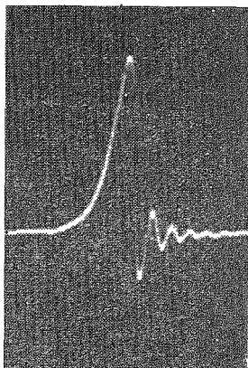
Рис. 9. Осциллограмма сигнала v(t) . Образец — 0,7 \text{ см}^3 одномолярного раствора \text{CuSO}_4 . Модуляция синусоидальная, амплитуда модуляции — 0,6 \text{ эрстед} , частота — 50 \text{ гц} . Полоса пропускания усилительного тракта от 20 \text{ гц} до 150 \text{ кгц} .
