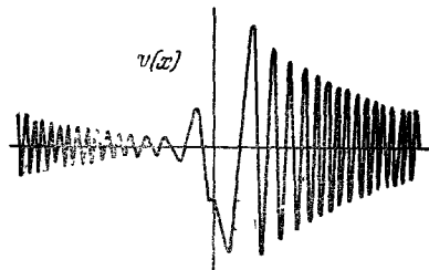
Рис. 6. График функции v(x) при синусоидальной модуляции продольной компоненты магнитного поля. Значения параметров те же, что и для рис. 5.
