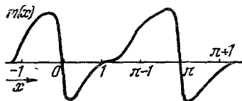
Рис. 8. Инверсия продольной компоненты результирующего вектора ядерного намагничивания. Значения параметров те же, что и для рис. 7.
