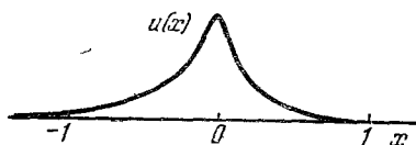
Рис. 7. График функции u(x) при наличии инверсии продольной компоненты результирующего вектора ядерного намагничивания. Значения параметров: \mu = 1 ; \nu = 0,1 ; k = 10 .
