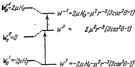
Рис. 13. Диаграмма сдвига энергетических уровней, обусловленного взаимодействием двух протонов в кристаллической решётке гипса.
