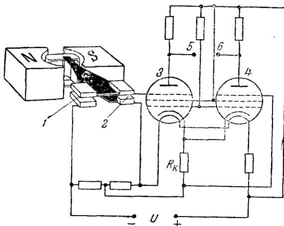
Рис. 19. \alpha -ионизационный стрелочный гальванометр и реле. 1 и 2 — ионизационные камеры.
