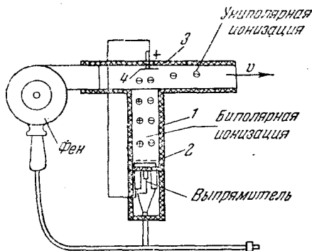
Рис. 13. Схема портативного радиевого аэроионизатора отрицательных ионов Н. И. Штейнбок.
