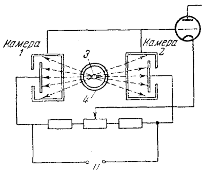
Рис. 22. Принципиальная схема \gamma -ионизационного способа измерения разностенности труб: 1 и 2 — ионизационные камеры, 3 — \gamma -излучатель, 4 — исследуемая труба.
