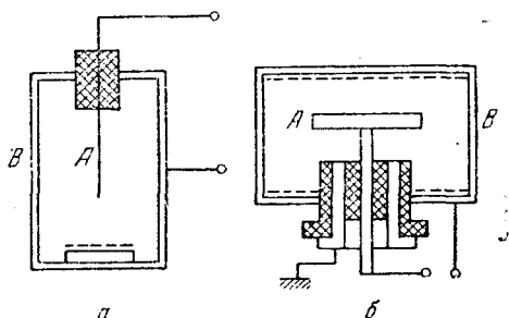
Рис. 4. Типичные конструкции цилиндрических ионизационных камер: a — без охранный кольца, б — с охранным кольцом.
