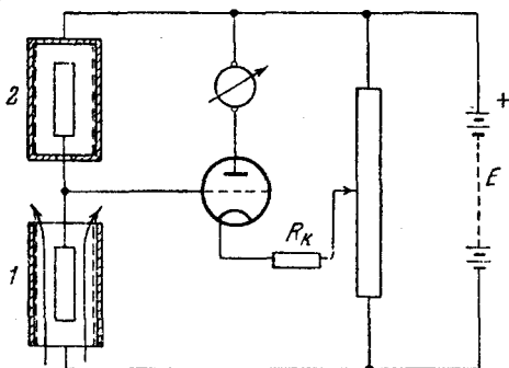
Рис. 9. Принципиальная схема \alpha -ионизационного газоанализатора. 1 и 2 — измерительная и эталонная камеры.
