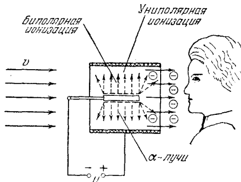
Рис. 12. Схема радиевого аэроионизатора отрицательных ионов А. Б. Вериги.
