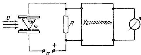
Рис. 11. Принципиальная схема \alpha -ионизационного измерителя скорости газового потока, основанного на уносе ионов потоком.
