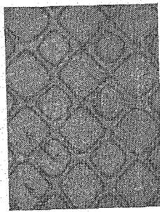
Рис. 5. Линии равной интенсивности второго порядка, полученные из рис. 4.
