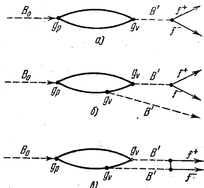
Рис. 5. Распад нейтрального бозона на пару частиц с полупелым спином (f^+, f^-) :
