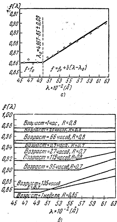
Рис. 1. Зависимость f(\lambda) для интерферометра Фабри-Перо с серебряными покрытиями в отражённом свете. а — пример экспериментального определения f(\lambda) для одного из случаев; б — зависимость f(\lambda) для слоёв с различной отражательной способностью и различного возраста.
