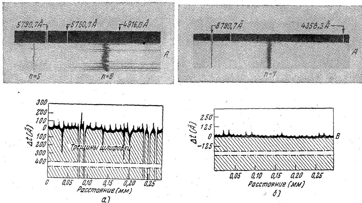
Рис. 2. Иррегулярности, наблюдаемые в полосах равного хроматического порядка, и их интерпретация. a — стеклянные поверхности, полированные в течение 20 минут; b — стеклянные поверхности, полированные в течение 450 минут.
