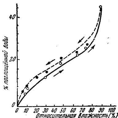
Рис. 3. Зависимость между количеством влаги, поглощенной сухой желатиной, и относительной влажностью 27 .
