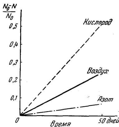
Рис. 4. Скорость поверхностной регрессии изображения в ядерных эмульсиях Илфорд С2, находящихся в различных газах при постоянной влажности 28 .
