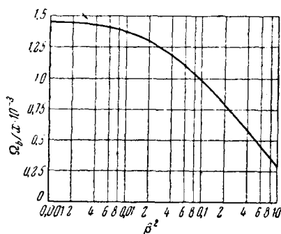
Рис. 24. Значение \frac{\Omega_b}{x} в зависимости от \beta^2 для однозарядных частиц в эмульсиях Ильфорд G5 87 .
