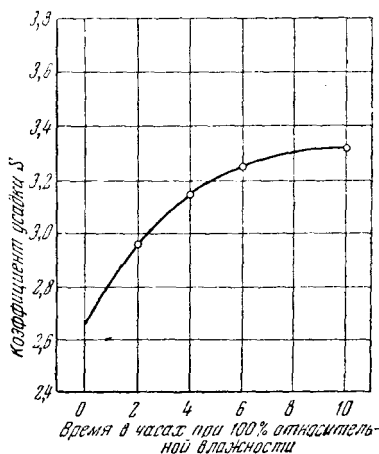
Рис. 30. Увеличение фактора усадки эмульсии Иلفорд G5 в зависимости от времени хранения при 100% относительной влажности III.
