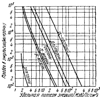
Рис. 18. Удельная потеря энергии различных частиц в ядерных эмульсиях в зависимости от их остаточного пробега. 10^4 \mu эмульсии \cong 4,0 \text{ г/см}^2 70 .
