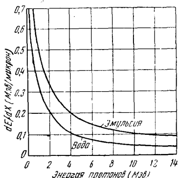
Рис. 15. Удельная потеря энергии протонов в зависимости от энергии в эмульсиях Ильфторд и в воде.
