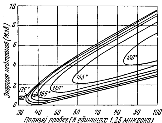
Рис. 34. Энергия нейтронов в зависимости от полного пробега в-эмульсии (в единицах 1,25 \mu ) \alpha -частицы и тритона, образованных при расщеплении \text{Li}^6 , для различных углов \theta ^{131} .
