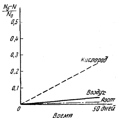
Рис. 5. Скорость внутренней регрессии изображения в ядерных эмульсиях Илфорд С2, находящихся в различных газах при постоянной влажности 28 .
