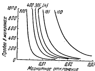
Рис. 37. Теоретические кривые пробег — кривизна в эмульсии Ильф-Форд С2 для однозарядных частиц различных масс 107 .
