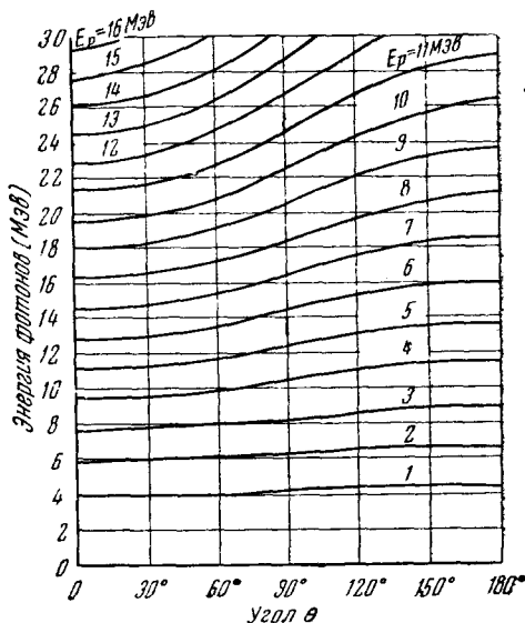
Рис. 35. Зависимость кинетической энергии протонов от энергии фотона и угла при фоторасщеплении дейтерона 67 .
