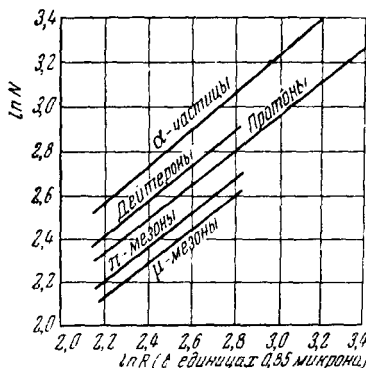
Рис. 17. Изменение полного числа зёрен N в зависимости от длины остаточного пробега R для следов различных частиц в эмульсиях Ильфорт С2, наполненных бором 69 .
