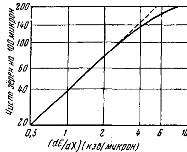
Рис. 8. Плотность зёрен в эмульсии Иلفорд G5 в зависимости от удельной потери энергии 47 .
