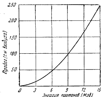
Рис. 10. Теоретическая кривая пробег — энергия для протонов в воздухе до энергии 15 Мэв 48 .
