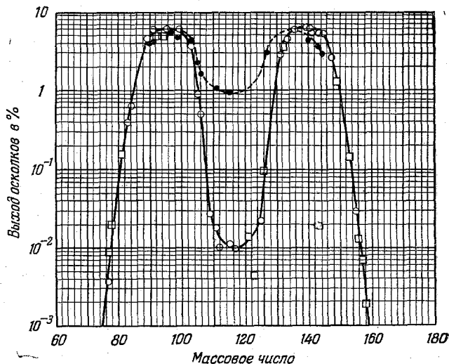
Рис. 46. Распределение масс осколков U^{235} при делении медленными нейтронами и нейтронами 14 Мэв.
