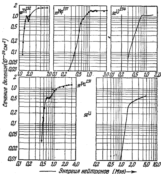
Рис. 43. Зависимость сечения деления нейтронами от энергии для пяти делящихся элементов 93 .
