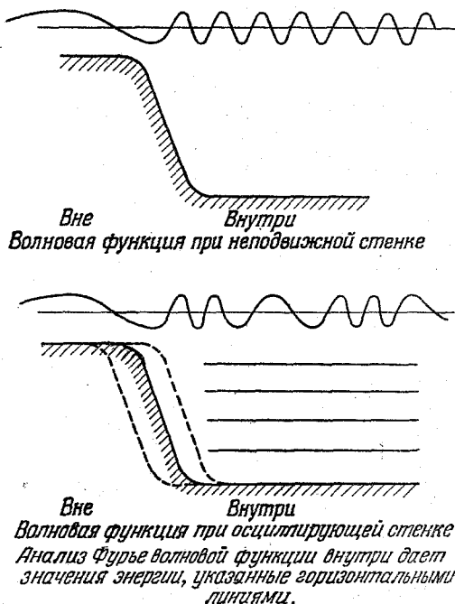
Рис. 39. Фазовая модуляция волновой функции нуклона вблизи ядерной поверхности.
