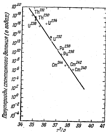
Рис. 45. Зависимость периодов спонтанного деления от \frac{Z^2}{A} .
