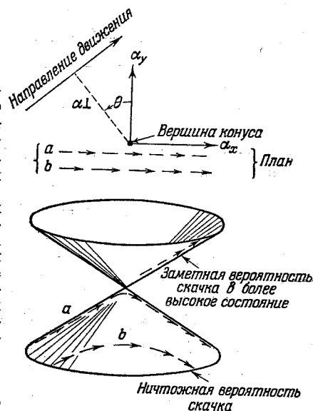
Рис. 35. Поперечное сечение перехода в случае конического контакта энергетических поверхностей.
