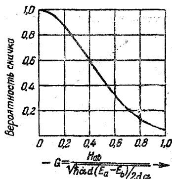
Рис. 34. Вероятность перехода из состояния \psi_a в состояние \psi_b в случае, когда деформационный параметр проходит вблизи точки пересечения \alpha_0 (рис. 33) с постоянной скоростью \dot{\alpha} 28.
