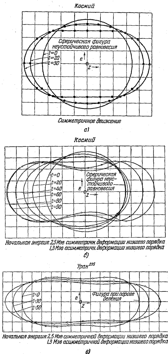
Рис. 51. Результаты динамического* анализа "ядерного деления, проведенного на основе модели жидкой капли ^{102} .
