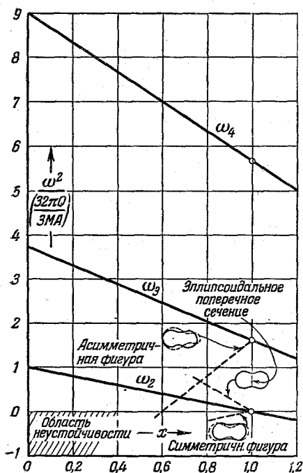
Рис. 48. Характеристические круговые частоты \omega колебаний низких порядков несжимаемой, равномерно заряженной жидкой капли с массой O и поверхностным натяжением O в зависимости от параметра делимости x . (В случае сферической фигуры — сплошные линии и в случае симметричной критической фигуры неустойчивого равновесия — пунктирные линии.)
