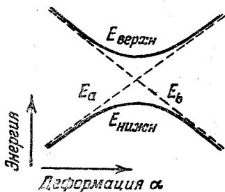
Рис. 33. Поведение двух уровней вблизи точки пересечения \alpha = \alpha_0 .
