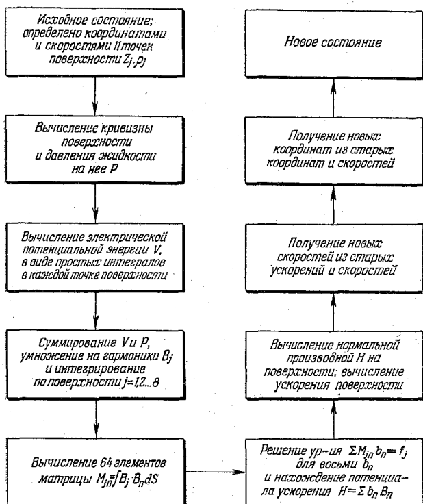
Рис. 52. Схема проведения гидродинамических расчётов рис. 51.
