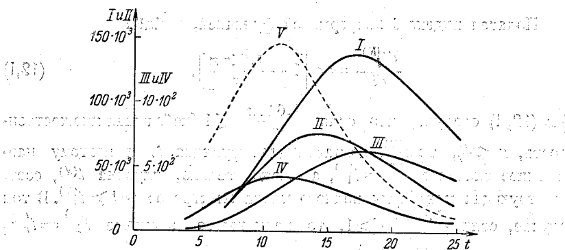
Рис. 5. Каскадные кривые. Кривые I и II описывают соответственно высотный ход электронной и ядерно-активной компонент, если n = 3 ; кривые III и IV — если n = 5 . Ординаты кривой V пропорциональны экспериментальным значениям 13 . По оси ординат левый масштаб соответствует числу электронов, а правый — числу ядерно-активных частиц.
