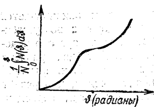
Рис. 3. Интегральное угловое распределение частиц в Ц-системе, полученное в 52 .
