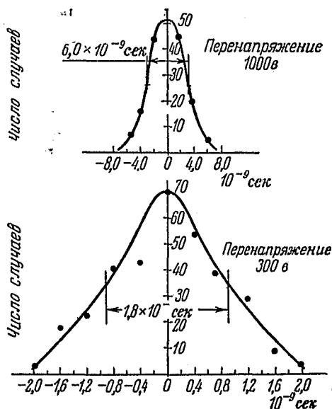
Рис. 2. Распределение запаздываний в искровом счётчике при перенапряжениях, равных 300 \text{ в} и 1000 \text{ в} .
