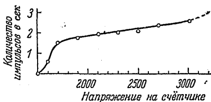
Рис. 1. Плато для счётчика, наполненного аргоном и кислотой. Время T_0 = 0,05 сек.
