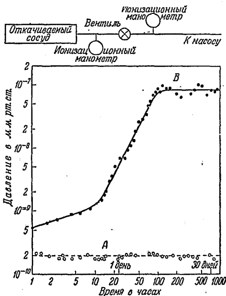
Рис. 3. Насыщение ионизационного манометра.
