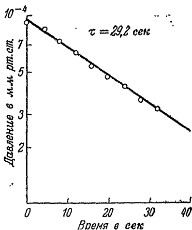
Рис. 2. Скорость откачки ионизационным манометром.
