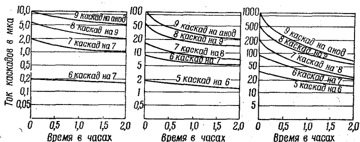
Рис. 13. Кривые утомления последних каскадов фотоумножителя при постоянном световом потоке, освещающем фотокатод.
