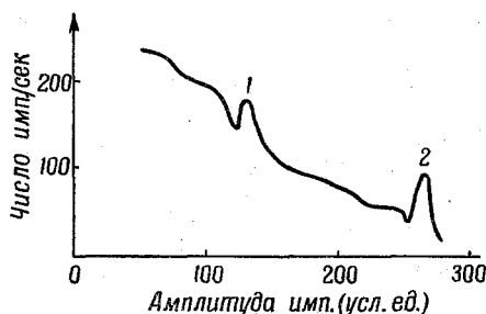
Рис. 30. Распределение интенсивности сцинтилляций в NaI·Tl; для \text{Na}^{24} максимум 1 соответствует энергии \gamma -лучей 1,4 Мэв, максимум 2 — 2,8 Мэв.
