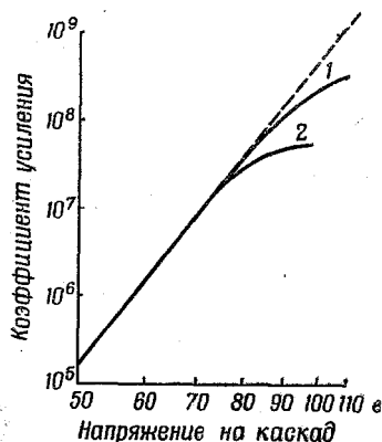
Рис. 12. Характеристика M = f(U_k) , построенная в логарифмическом масштабе по обеим осям. Загиб характеристики вызван влиянием объёмного заряда в анодной части фотоумножителя: 1 — анодное напряжение 200 в, 2 — анодное напряжение 100 в.
