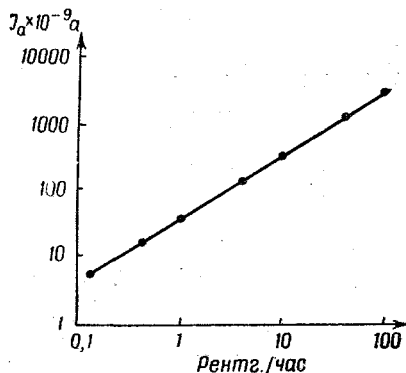
Рис. 32. Зависимость анодного тока фотоумножителя 1P21 от интенсивности лучей от радиового источника, воздействующих непосредственно на фотокатод фотоумножителя.
