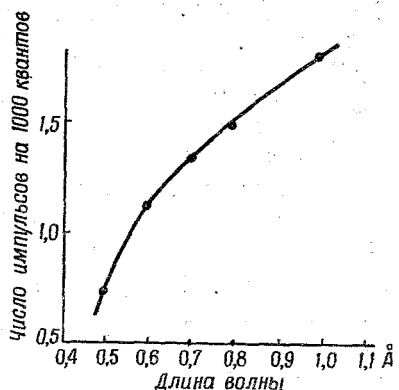
Рис. 36. Зависимость числа импульсов на каждую тысячу квантов от длины волны рентгеновских лучей в электронном умножителе с танталовым катодом.
