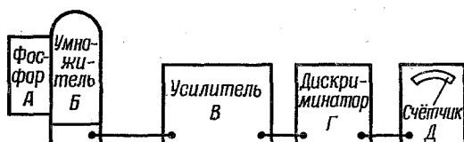
Рис. 1. Блок-схема сцинтилляционного счётчика.
