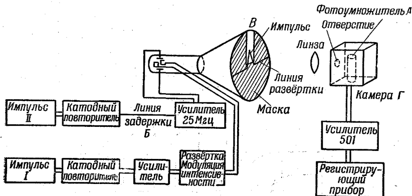
Рис. 20. Схема совпадений с большой разрешающей способностью.
