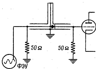
Рис. 17а. Схема формирования импульса фотоумножителя с помощью короткозамкнутой линии задержки.
