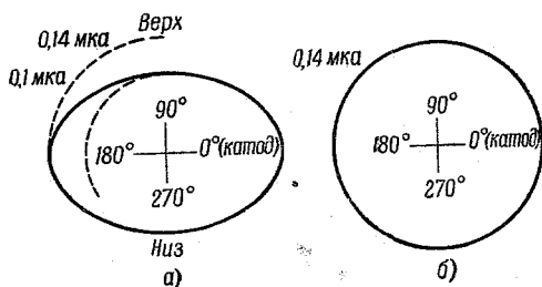
Рис. 33. Кривые направленности чувствительности фотоумножителя 1P21 к \gamma -излучению.
