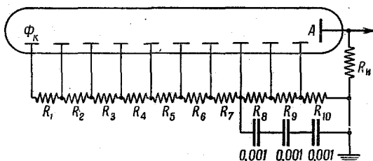
Рис. 15а. Схема включения фотоумножителя.
