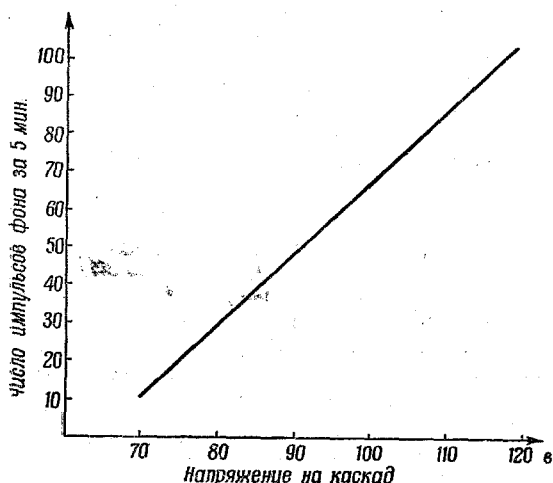
Рис. 6. Зависимость фона от напряжения для охлажденного фотоумножителя 1P21.
