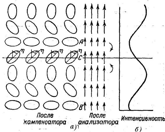
Рис. 2. Вращение эллипса поляризации компенсатором (а) и изменение интенсивности света, проходящего через анализатор (б), в функции расстояния от центрального сечения компенсатора.
