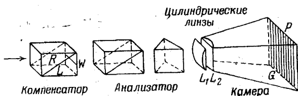
Рис. 1. Оптическая схема установки.
