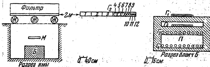
Рис. 13. Схема установки для исследования свойств ядерно-активной компоненты широких атмосферных ливней. Счётчики М срабатывают от частиц электронно-ядерных ливней, образованных в фильтре. Блок Б служит для определения плотности ливней, а годоскопическая группа счётчиков — для определения плотности атмосферных ливней.
