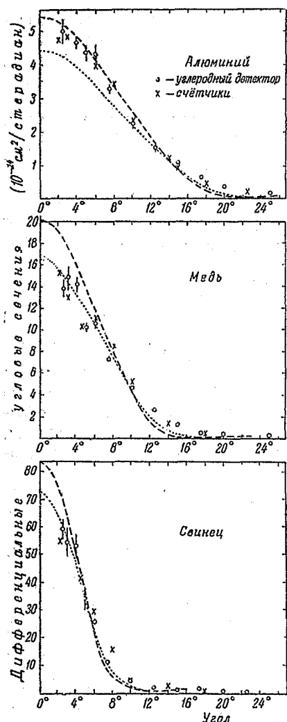
Рис. 35. Дифракционное рассеяние нейтронов с энергией 84 Мэв на алюминии, меди и свинце. Крупный пунктир соответствует расчёту по интегральным сечениям упругого рассеяния, полученным интегрированием дифференциальных сечений. Мелкий пунктир соответствует расчёту по интегральным сечениям упругого рассеяния, полученным из разности полных сечений и сечений неупругих столкновений.
