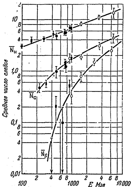
Рис. 42. Зависимость среднего числа следов различной ионизации от кинетической энергии частиц, образовавших звезду (● — для звёзд от протонов, 8 — для звёзд от \pi -мезонов, ○ — для звёзд от ( \pi , p)-частиц).
