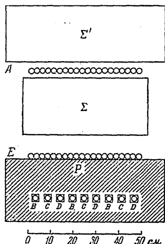
Рис. 44. Схема одной из установок для измерения среднего пути взаимодействия частиц, генерирующих электронно-ядерные ливни.
