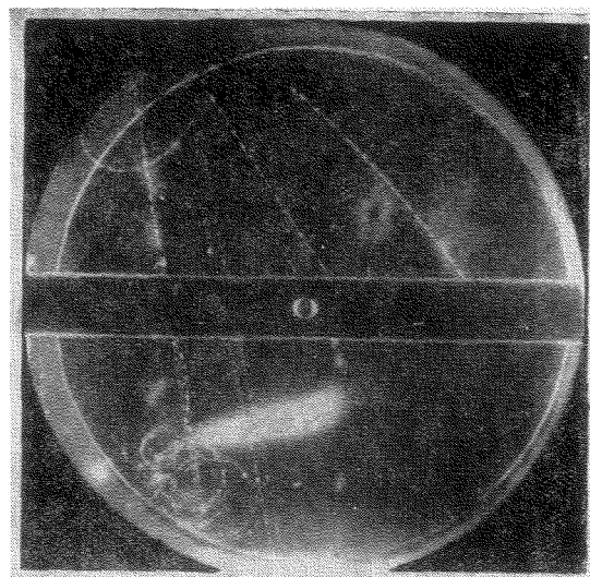
Фотография VIII (см. § 3.1). Вторичная частица, возникшая при распаде нейтральной V -частицы, является отрицательно заряженным \pi -мезоном. Отрицательно заряженная частица (1) имеет импульс 82 \text{ Мэв/с} ( \pm 5\% ) и ионизацию, в 2, 5—3,5 раза превышающую минимальную. \pi -мезон с таким импульсом обладал бы трёхкратной ионизацией. След положительно заряженной частицы направлен в сторону поршня камеры и поэтому быстро выходит из поля зрения. Угол между направлениями движения вторичных частиц равен 27^\circ .
