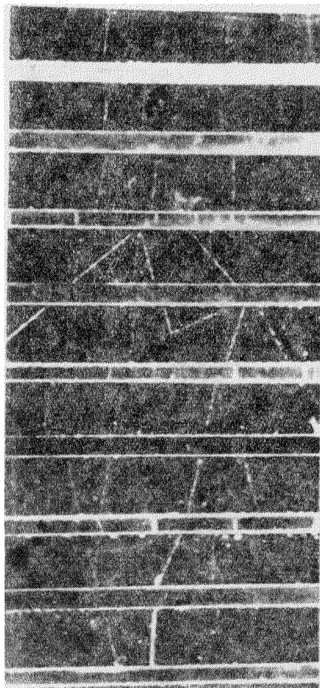
Фотография XIV (см. § 11.4). Распад медленной V-частицы. Медленная заряженная частица распадается между 4 и 5 пластинами. В камере помещено попеременно 8 алюминиевых и свинцовых пластин. Вторичная частица создаёт ионизацию, в два раза превышающую минимальную, и направление её движения составляет угол 90^\circ с направлением движения V-частицы. Затем вторичная частица попадает в алюминиевую пластину, расположенную над точкой распада. Авторы предполагают, что здесь она рассеивается на большой угол, после чего движется вниз и останавливается, пройдя четыре пластины. По наблюдаемым значениям пробега, рассеяния и ионизации они заключают, что эта частица является мезоном, и так как частица испытывает ядерное рассеяние, то, вероятно, это \pi -мезон.
