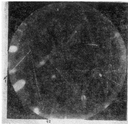
Фотография VII (см. §§ 3.1 и 6.1). Распад нейтральной V -частицы на протон и мезон. V -образный след образован следами (1) и (2), угол между которыми равен 50,5^\circ . Ионизация вдоль следа (1) равна (3—4) от минимальной ионизации. Импульс частицы (1) равен 0,48 \text{ Бэв/с} . Со значительной достоверностью эта частица должна быть признана протоном. Отрицательно заряженная частица имеет импульс 0,19 \text{ Бэв/с} и вероятно, что это \pi -мезон. V -образный след может быть объяснён такой схемой распада:
