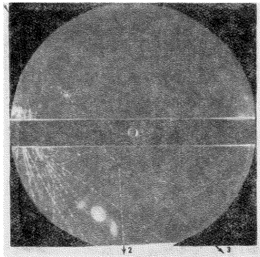
Фотография XI (см. § 4.1). Ядерное взаимодействие в газе. Взаимодействие возникло под пластиной и было вызвано частицей (1). Между образовавшимися при этом следами (2) и (3) виден сгусток ионизации, образованный, повидимому, ядром отдачи. След (1) не может быть промерен, так как он частично закрыт следом \delta -частицы малой энергии. Измеренный импульс положительно заряженной частицы (2) равен 0,35 \text{ Бэв/с} , а ионизация вдоль следа (2) превышает минимальную в 4—5 раз; повидимому, частица (2) есть протон. Измеренный импульс положительно заряженной частицы (3) равен 0,65 \text{ Бэв/с} и след этой частицы наклонён под углом, близким к 7^\circ к плоскости следов (1) и (2). В направлении, составляющем прямой угол с направлением первичной частицы (1), закон сохранения импульса не выполняется. Поэтому этот случай не может быть просто упругим рассеянием.
