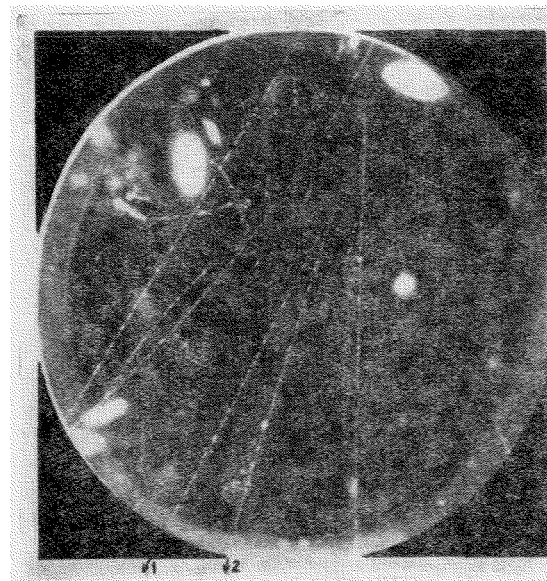
Фотография XII (см. § 6.1). V-образный след большой энергии с малым углом разлёта. Вилка образована двумя следами (1) и (2) большой энергии, расходящимися под углом 12^\circ . Измеренные импульсы положительно (1) и отрицательно (2) заряженной частицы равны соответственно 1,5 \text{ Бэв/с} и 1,6 \text{ Бэв/с} . Подробное рассмотрение динамики распадных процессов приводит к заключению, что в данном случае, вероятно, имеет место распад, происходящий по схеме:
