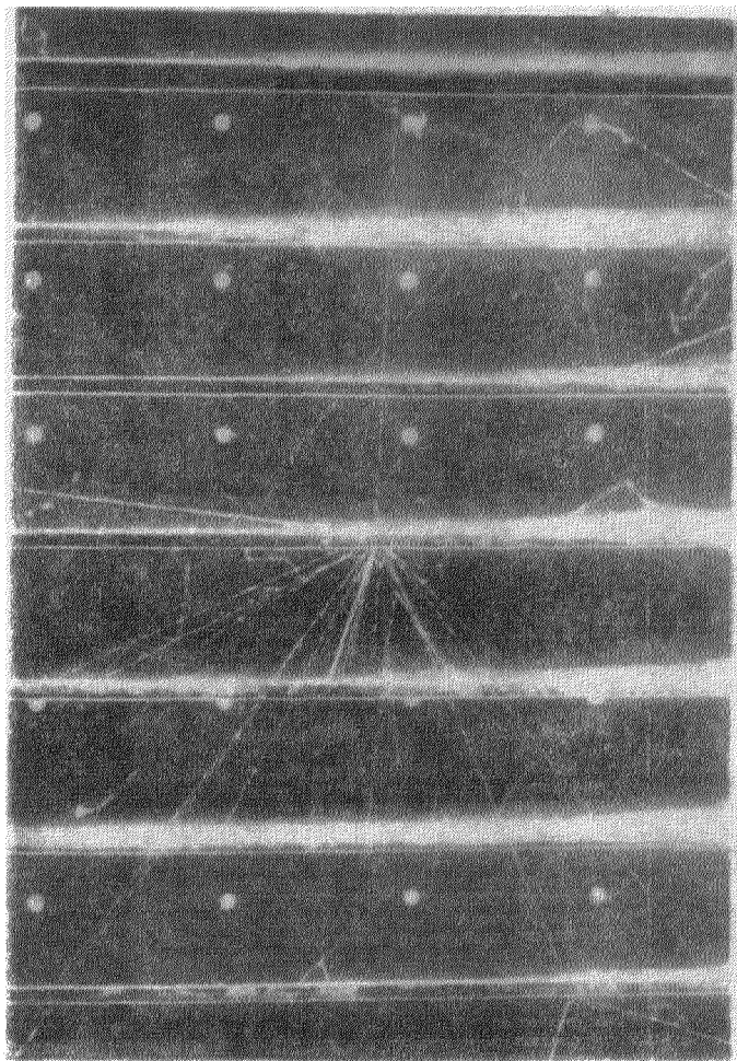
Фотография IV (см. § 2.3). Рождение нейтральной V -частицы. В четвертой пластине возникло ядерное взаимодействие большой энергии. Между четвертой и пятой пластинами виден V -образный след, образованный двумя частицами, из которых одна создает сильную ионизацию. Ионизация от другой частицы минимальная. Медленная частица поглощается в пятой пластине. Тонкий вторичный след проникает до седьмой пластины, испытывая заметное рассеяние в шестой. Из описания V -образного следа по отношению к точке зарождения V -частицы можно заключить, что импульс медленной частицы больше импульса проникающей вторичной частицы. Весьма вероятно, что медленная частица — протон, а другая вторичная частица — мезон.
