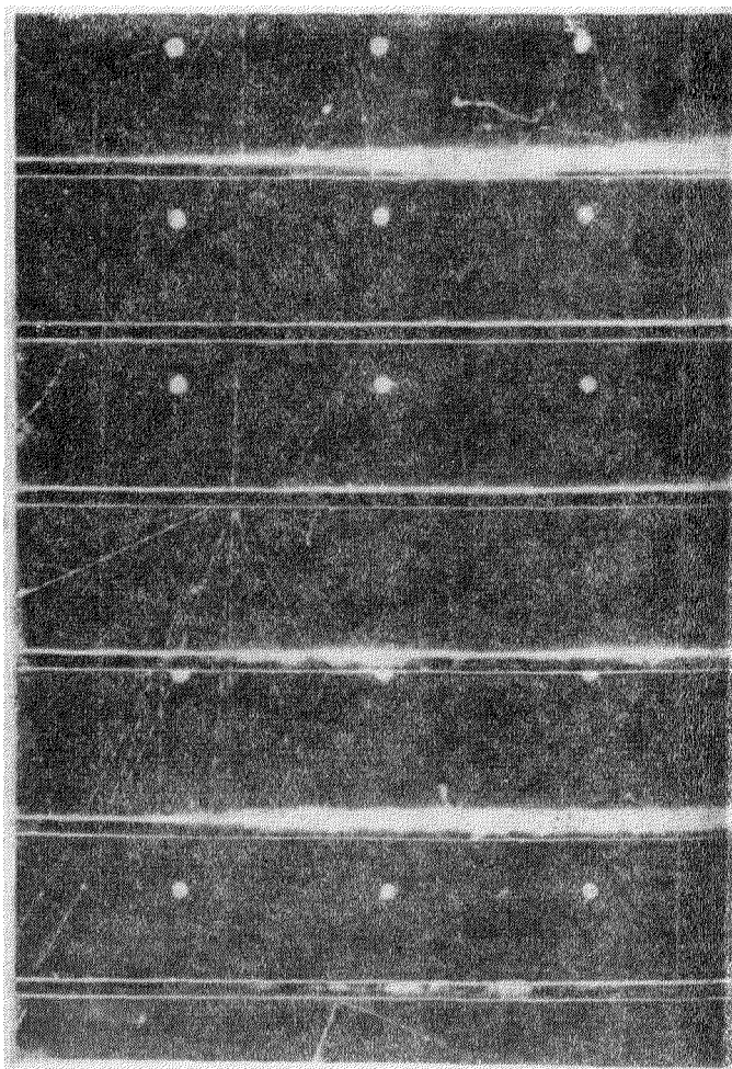
Фотография III (см. § 2.3). Рождение нейтральной V -частицы. Заряженная частица создала в третьей свинцовой пластине ядерное взаимодействие большой энергии. V -образный след расположен между третьей и четвертой пластинами. Длина пути нейтральной V -частицы, по видимому, меньше 2 см. Обе вторичные частицы создают минимальную ионизацию. Правая частица проходит по меньшей мере две пластины и сильно рассеивается в четвертой пластине.
