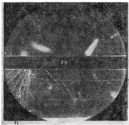
Фотография XVI (см. § 11.5). Распад медленной отрицательно заряженной V -частицы. В ядерном взаимодействии большой энергии, которое произошло в свинцовой пластине, возникла медленная V -частица, распавшаяся на расстоянии 2 см под пластиной. Из-за малой длины первичный след не может быть промерен, но всё же видно, что ионизация превышает минимальную в четыре раза. След отрицательно заряженной частицы (2) образует угол 100^\circ с направлением первичной частицы. Измеренный импульс частицы (2) равен 0,18 \pm 0,02 Бэв/с. Минимальное и максимальное значения массы отрицательно заряженной V -частицы могут быть вычислены: они приведены в таблице XI § 11.5. Если, например, нейтральная вторичная частица есть \pi -мезон, то масса V -частицы лежит между 900 m_e и 1080 m_e , если же нейтральная частица есть V -частица с массой 800 m_e , то масса V -частицы лежит между 1310 m_e и 1440 m_e .
