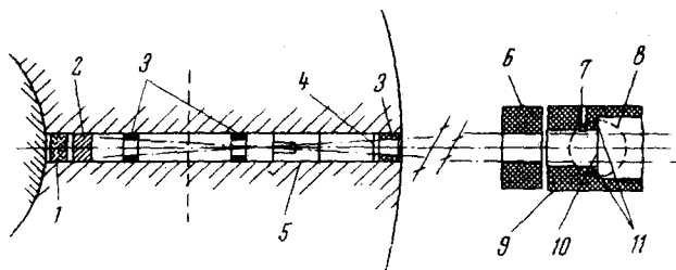
Рис. 10. Схема гамма-спектрометра: 1 — вискмутый экран; 2 — мишень; 3 — внутренние свинцовые диафрагмы; 4 — кадмиевый экран; 5 — пробка из бора и парафина; 6 — свинцовая входная диафрагма; 7 — катушка магнетометра; 8 — полюсы электромагнита; 9 — свинцовый кожух; 10 — радиатор; 11 — счётчики.
