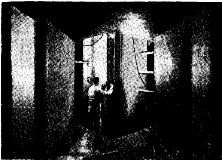
Рис. 4. Отверстие в защите, которое занимает термическая колонка; видны реакторный бак, трубы для облучения и одна из кадмиевых пластин.
