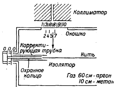
Устройство счётчика с корректирующей трубкой.
