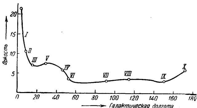
Распределение инфракрасной яркости по протяжению Млечного Пути. I— \alpha -Змееносца, II— \delta -Орла, III— \gamma -Орла, IV— \beta -Лебеда, V— \gamma -Лебеда, VI— \alpha -Лебеда, VII— \gamma -Кассиопея, VIII— \alpha -Персея, IX— \beta - \xi -Тельца, X— \epsilon -Ориона.
