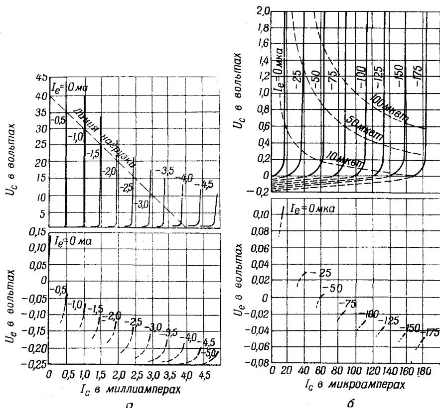
Рис. 2. Статические характеристики кристаллического триода типа n-p-n . а) — при сравнительно больших токах; б) — при очень малых токах.
