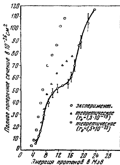
Рис. 2. Сравнение суммы поперечных сечений реакций (p, n), (p, 2n) и (p, pn) на \text{Cu}^{63} в функции энергии протонов с теоретически рассчитанными сечениями поглощения протона ядром \text{Cu}^{63} .
