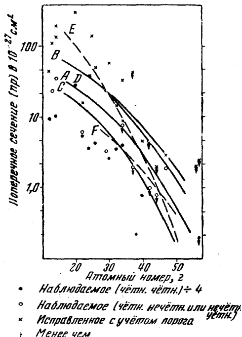
Рис. 3. Поперечное сечение (n, p) реакции в функции Z . Сплошные линии — теоретические кривые — А: r_0 = 1,3 \cdot 10^{-13} \text{ см} и T из работы V. Weisskopf, Lecture Series in Nuclear Physics (U. S. Govt Printing Office, Washington D. C., 1947); В: r_0 = 1,5 \cdot 10^{-13} \text{ см} ; С: r_0 = 1,3 \cdot 10^{-13} \text{ см} , T' = 0,75 \text{ Г} ; Д: r_0 = 1,3 \cdot 10^{-13} \text{ см} , T'' = 1,25 \text{ Г} ; Е: r_0 = 1,3 \cdot 10^{-13} \text{ см} , T из работы V. Weisskopf and J. M. Blatt (не опубликовано) по данным работы 10 .
