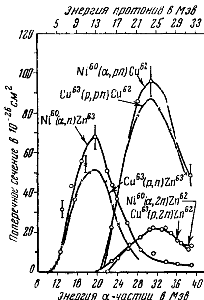
Рис. 1. Экспериментальные поперечные сечения для (pn), (p, 2n), (p, pn) реакций на \text{Cu}^{63} и для ( \alpha, n ), ( \tau, 2n ) и ( \alpha, pn ) реакций на \text{Ni}^{60} в функции энергии протонов и \alpha -частиц соответственно.
