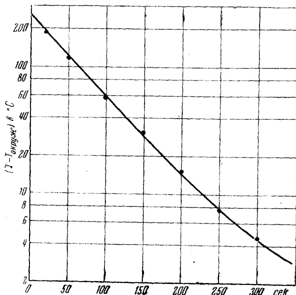
Рис. 13. Характеристика охлаждения массивного термистора: \lg(T - T_{\text{окрж}}) как функция времени.
