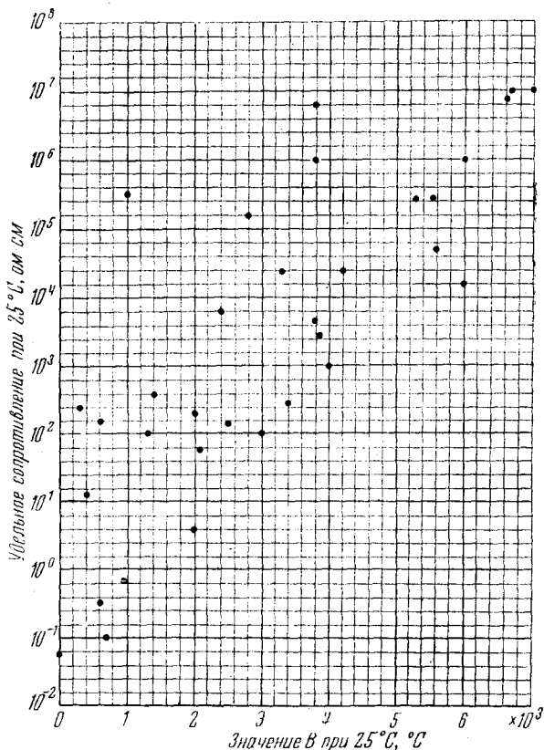
Рис. 7. График зависимости \lg \rho от V для различных полупроводников. (Величина V — согласно уравнению (4) — пропорциональна температурному коэффициенту сопротивления \alpha .)
