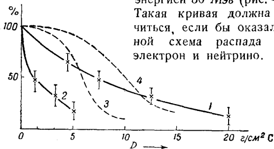
Рис. 47. Кривые поглощения электронов распада в фильтре D : 1 — экспериментальная кривая поглощения в свинце; 2 — кривая поглощения в графите; 3 — расчёт поглощения в графите в предположении, что все электроны распада имеют энергию 25 Мэв; 4 — расчёт поглощения в графите в предположении, что все электроны распада имеют энергию 50 Мэв.
