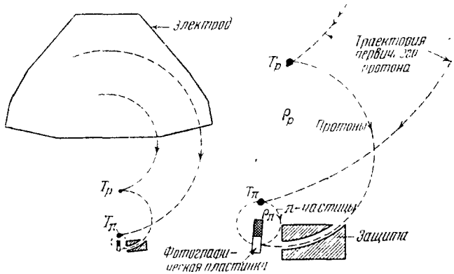
Рис. 12. Установка 88 для определения массы \pi^+ -мезонов по методу Д. Две мишени T_p и T_\pi служат источником протонов и \pi -мезонов. Радиусы \rho_p и \rho_\pi относятся приблизительно как массы:
