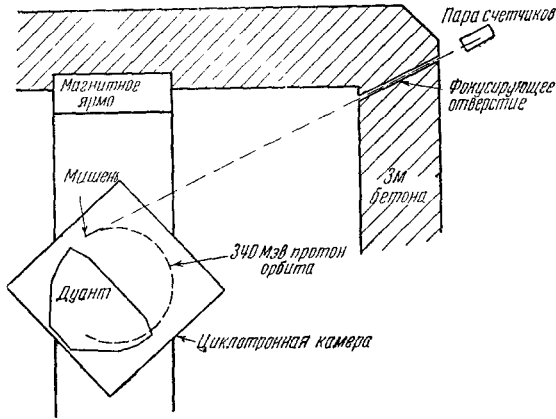
Рис. 32. Расположение аппаратуры для наблюдений \gamma -излучения, образованного при столкновении 340-МэВ протонов с веществом.
