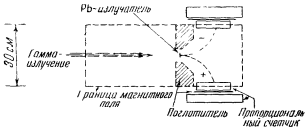
Рис. 33. Аппаратура для определения интенсивности \gamma -лучей и энергии фотонов 102 .
