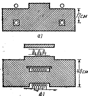
Рис. 26. Установки 87, 88 для наблюдения ливней проникающих частиц.
