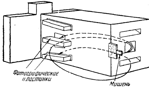
Рис. 14. Установка Ричардсона 43 для определения времени жизни \pi -мезонов, искусственно полученных в синхроциклотроне. При отсутствии распада число частиц на единицу площади каждой пластинки (без учёта автофазировки) обратно пропорционально длине пути до соответствующей пластинки. Не показана траектория бомбардирующего пучка \alpha -частиц.
