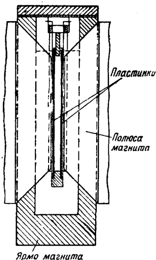
Рис. 7. Установка, использованная Францинетти для определения массы частиц космических лучей в опытах по магнитному отклонению. Метод В.
