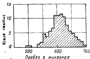
Рис. 2. Распределение значений пробегов в эмульсии Иلفорд С2 для 90 \mu^+ -частиц, образованных при распаде \pi^+ -частиц, остановившихся в эмульсии. Наблюдаемое распределение согласуется с ожидаемым для частицы с постоянной скоростью из-за флуктуаций в пробегах и доказывает, что \pi^+ -частицы обычно обладают весьма малой скоростью в момент распада. Среднее значение пробега \approx 612 \mu ; соответствующее значение кинетической энергии E_\mu = 4,15 \text{ Мэв} .
