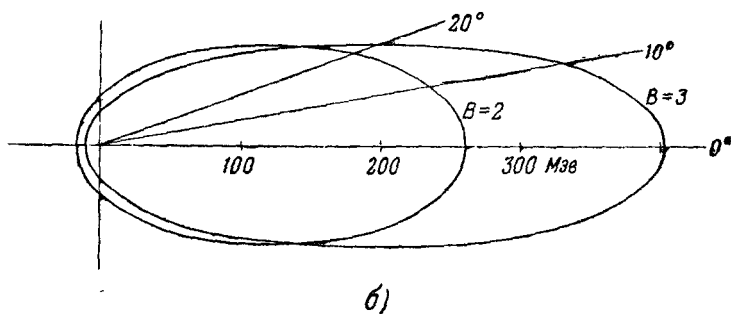
Рис. 31. Характеристики излучения, образованного при распаде нейтрального мезона: а) энергетический спектр фотонов, образованных моноэнергетическим пучком нейтральных мезонов; б) энергия фотонов как функция угла вылета. Кривые даны для различных значений B , причём Bm_0c^2 — суммарная энергия частицы с массой покоя m_0 .
