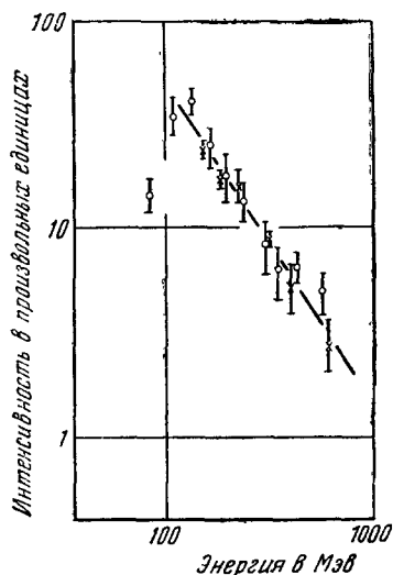
Рис. 36. Энергетическое распределение заряженных (кружки) и нейтральных (крестики) \pi -мезонов в атмосфере на высоте 21 км. Интенсивность отложена в произвольных единицах.
