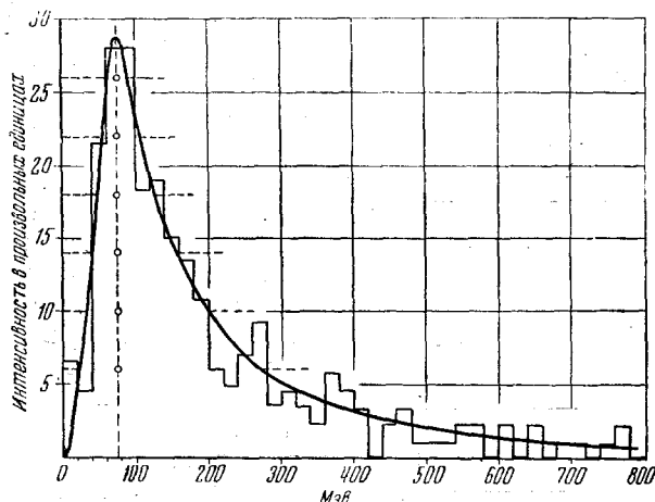
Рис. 35. Спектр \gamma -лучей в воздухе на высоте 21 км 103 .
