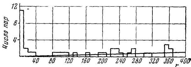
Рис. 38. Определение времени жизни нейтральных мезонов. Величина r — перпендикуляр, опущенный из «звезды» на биссектрису угла между линиями движения электронов пара. Концентрация случаев, для которых r < 40 \mu , вызывается «связанными» парами. Такие случаи доказывают, что \gamma -лучи образуются в ядерных взрывах и позволяют определить интенсивность таких \gamma -лучей.
