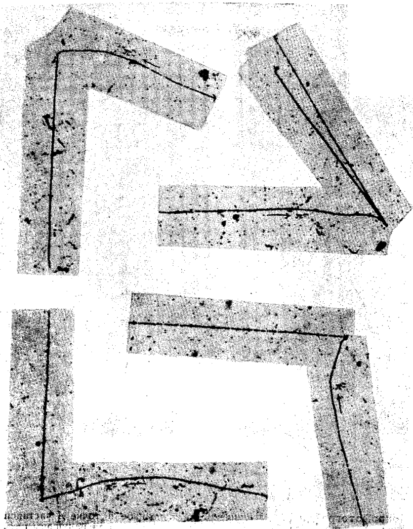
Микрофотография III. Расщепление ядер тяжёлых элементов при захвате \pi -частиц.
