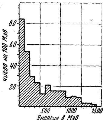
Рис. 28. Распределение по энергиям мезонов, входящих в состав ливней, наблюденное на высоте 21 км.
