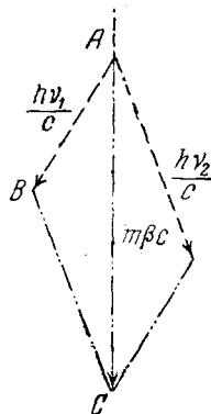
Рис. 30. Баланс импульсов при распаде нейтрального мезона на два кванта.
