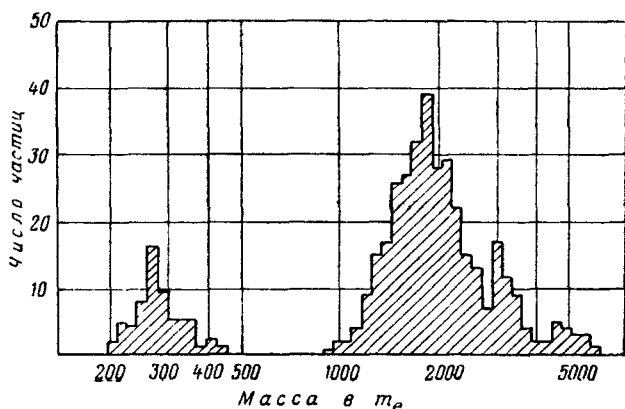
Рис. 11. Распределение значений (определённых по методу Г) масс частиц, испущенных в звёздах 81 .
