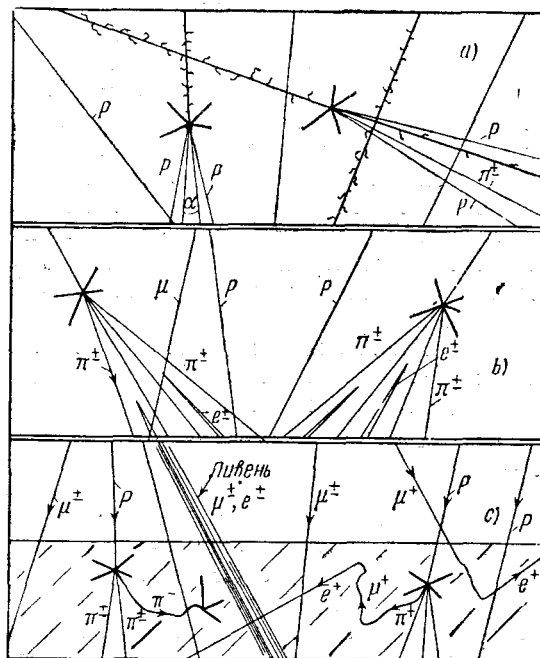
Рис. 42. Схематическое изображение процессов, происходящих в атмосфере.
