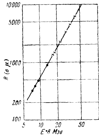
Рис. 3. Зависимость между \ln R (пробег в микронах) и \ln E (энергия в Мэв) для протонов в эмульсии Ильфорд С2 (Латтес, Фаулер, Кур 8 , Баркас, Бишоп, Браннер 32 ). Прямая линия соответствует равенству
