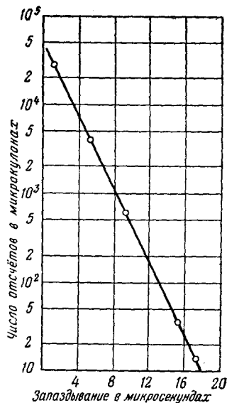
Рис. 19. Данные по запаздыванию моментов распада искусственно образованных \mu^+ -мезонов 73 .
