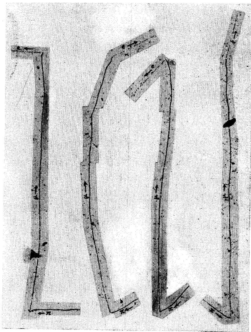
Микрофотография I. Четыре примера последовательного \pi - e -распада. Отчётливо видно увеличение плотности зёрен на конце пробега \mu -мезона, а также малая плотность зёрен в следах электронов.
