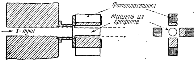
Рис. 25. Схема установки для изучения образования мезонов \gamma -лучами больших энергий 83 . Распределение \pi^+ и \pi^- -мезонов по энергиям определялось по суммарной толщине поглотителя, которую должны пройти мезоны до остановки в фотографической эмульсии 82 .
