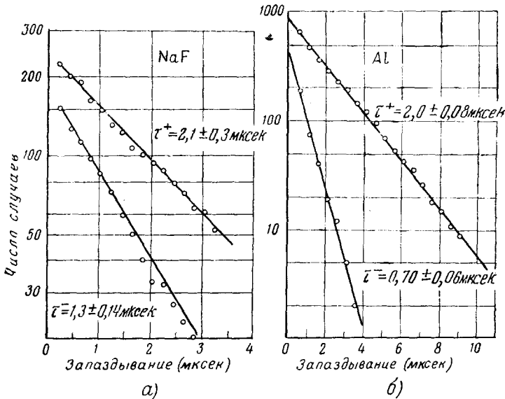
Рис. 20. Распад \mu^- -мезонов в NaF и в Al.
