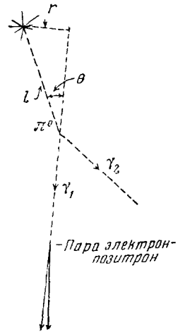
Рис. 37. Принцип метода определения времени жизни нейтральных мезонов.
