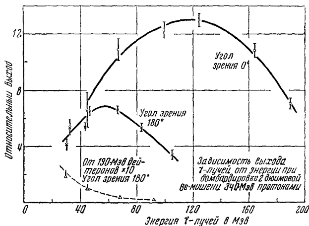
Рис. 34. Характеристики излучения, образованного при бомбардировке углерода 340-Мэв протонами. Показано спектральное распределение для двух направлений испускания фотонов относительно линии движения генерирующих частиц.
