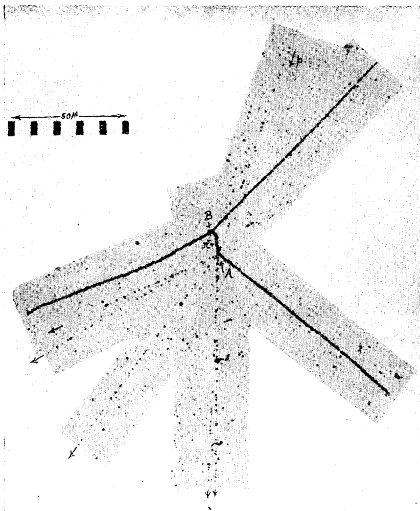
Микрофотография IV. Расщепление, образованное в точке A частицей (след p ), движущейся с релятивистской скоростью. Были испущены пять быстрых ливневых частиц и отрицательный \pi -мезон. Последний останавливается в точке B и образует вторичное расщепление. Кроме того, испущена одна неидентифицированная сильно ионизирующая частица, вероятно протон.
