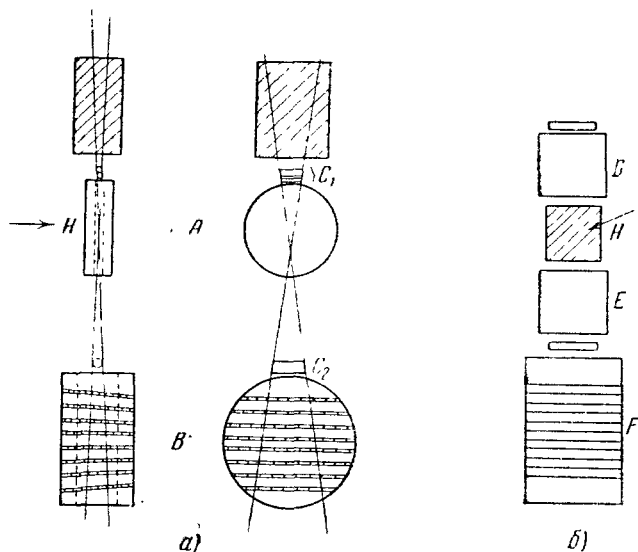
Рис. 9. Установка а) Фреттера и б) Броде для определения массы частиц космических лучей. В установке Фреттера две камеры Вильсона А и В одновременно срабатывают при разрядах в управляющих счётчиках C_1 и C_2 . Верхняя камера помещена в магнитное поле \sim 5000 гаусс и служит для измерения импульса частиц, останавливающихся в свинцовых пластинках в нижней камере. В установке Броде импульс измеряется с помощью двух камер Вильсона D и E, разделённых областью H, в которой постоянным магнитом создаётся магнитное поле. Изменение в направлении движения частицы в магнитном поле, определённое по следу в обеих камерах, даёт значение её импульса. Частица останавливается в одной из свинцовых пластинок в третьей камере Вильсона.
