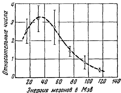
Рис. 23. Энергетический спектр искусственных мезонов, образованных протонами.
