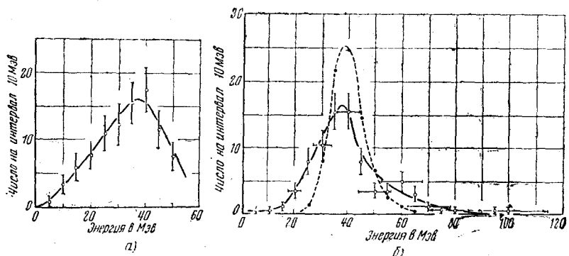
Рис. 17. а) Распределение по энергиям электронов, образованных при распаде \mu^- -мезонов. Измерения Андерсона и др. б) Распределение по энергиям электронов, образованных при распаде \mu^- -мезонов. Измерения Дэвиса и др. Пунктирная кривая соответствует распределению, ожидаемому для моноэнергетической группы электронов с энергией 40 Мэв.
