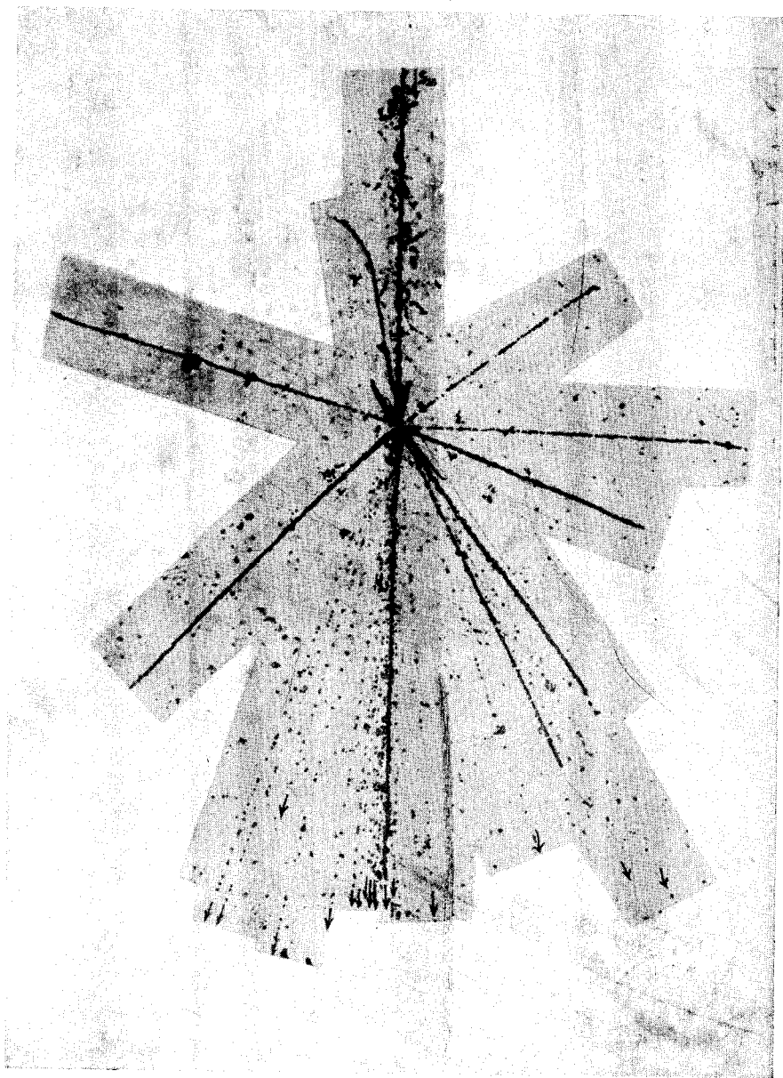
Микрофотография XII. Ядро серы ( Z = 16 \pm 1 ) сталкивается в эмульсии с ядром серебра или брома. В результате столкновения образуется ядро фтора и 25 ливневых частиц — протонов, \pi -мезонов.
