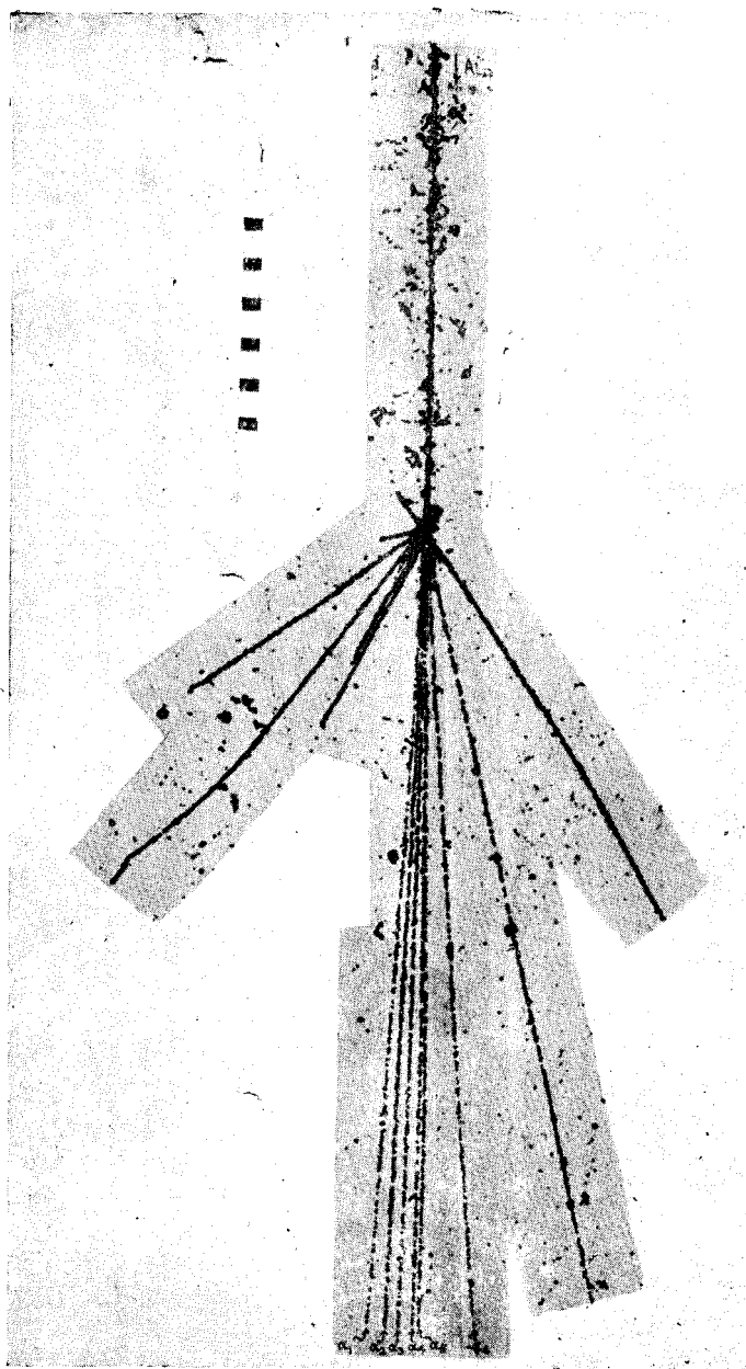
Микрофотография IX. Ядро алюминия ( Z = 13 \pm 2 ) испытывает соударение, в результате которого испускаются шесть \alpha -частиц, движущихся внутри узкого конуса с примерно равными скоростями. Возможно что они принадлежат первичному ядру.
