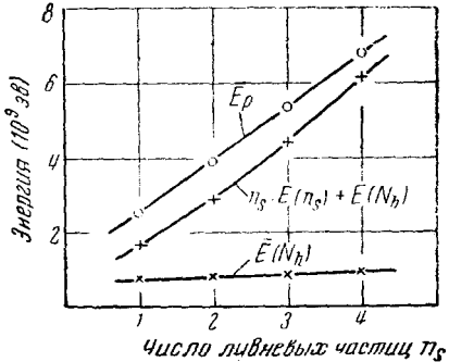
Рис. 29. Энергетический баланс звёзд с различным числом частиц: \bar{E}_p — средняя энергия первичного протона; n_s \bar{E}_s — среднее значение суммарной энергии ливневых частиц и \bar{E}(N_h) — средняя энергия звезды. Легко видеть, что нехватает некоторой доли энергии; предполагается, что эта энергия была затрачена на образование нейтральных мезонов.
