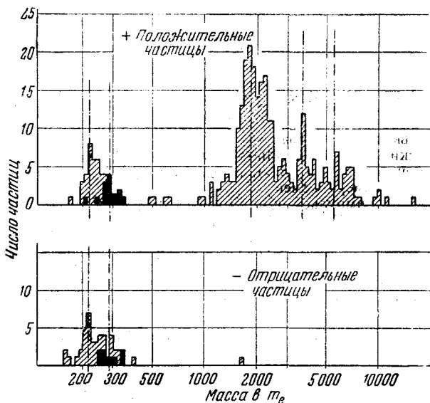
Рис. 8. Распределение значений масс положительных и отрицательных частиц в космических лучах на высоте 3400 м. Результаты показывают, что частицы с массой \sim 1000 m_e существуют в количестве, не большем, чем 5% от числа \pi -и \mu -мезонов. Чёрные квадраты относятся к \pi^+ - и \pi^- -мезонам, идентифицированным по вторичным эффектам, наблюдаемым на конце их пробега.
