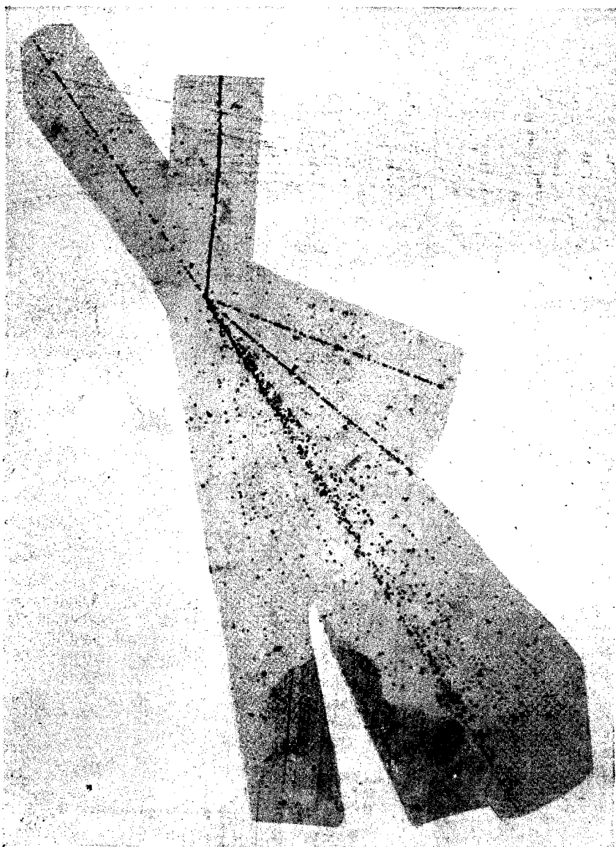
Микрофотография VIII. \alpha -частица большой энергии, след которой виден в левом верхнем углу микрофотографии, взаимодействует с ядром и образует 35 ливневых частиц, большинство из которых движется в узком конусе.
