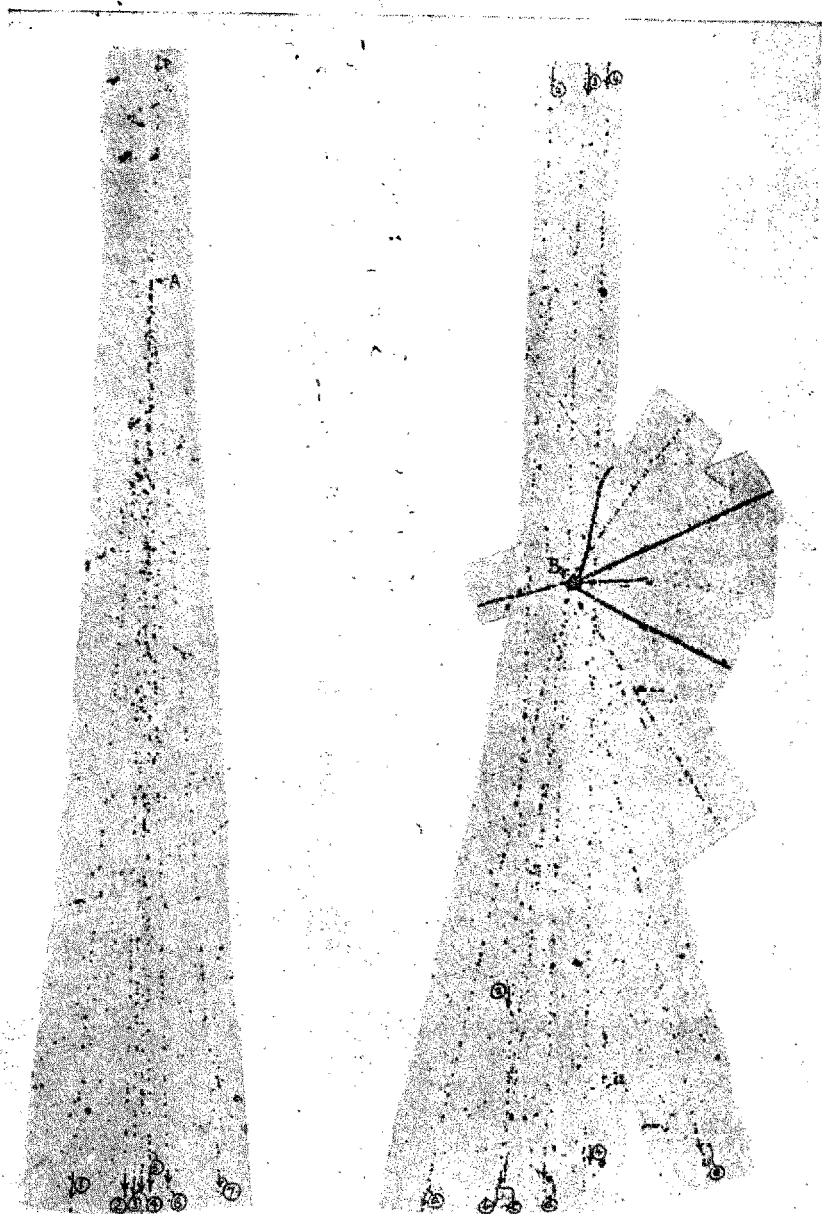
Микрофотография VII. В результате ядерного столкновения в точке А быстрая частица (след P ) образовала ливень из семи частиц. Ливневая частица 3 создала вторичный ливень в точке В. Ливень в точке А создаётся, возможно, в результате взаимодействия протона с протоном.
