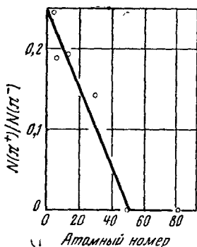
Рис. 24. Отношение числа положительных мезонов к отрицательным \frac{N(\pi^+)}{N(\pi^-)} в энергетическом интервале от 2 до 5 Мэв; мезоны образовались при столкновении 390-Мэв \alpha -частиц с ядрами, имеющими различный атомный номер 82 .
