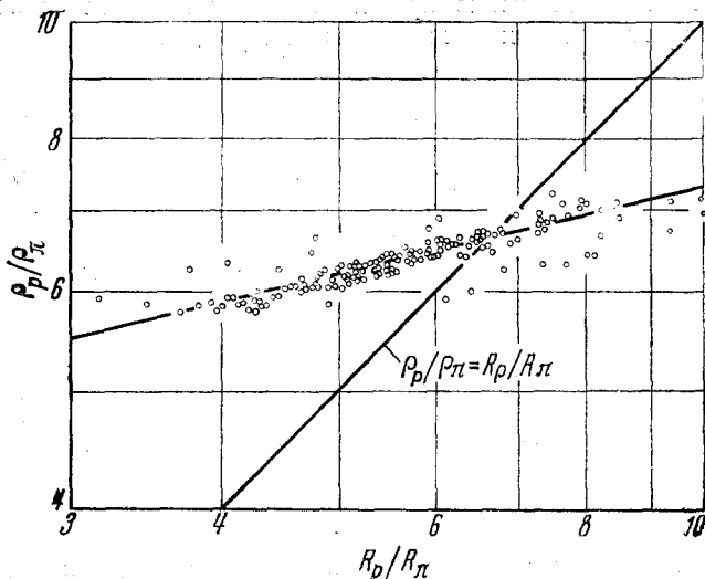
Рис. 13. Зависимость \frac{R_p}{R_\pi} для следов индивидуальных
