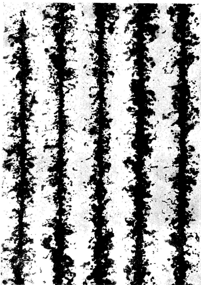
Микрофотографии X—XI. Последовательные участки следа ядра железа наливается в правом нижнем. Обрыв в следе между участками 7 и 8 еиями. Хорошо видно уменьшение пробегов \delta -электронов с уменьшением электронов
