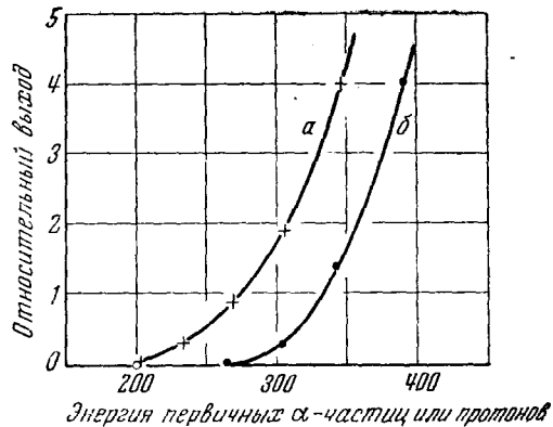
Рис. 21. Зависимость выхода \pi -мезонов, как функция энергии первичной частицы; кривая a — протоны; кривая b — \alpha -частицы.
