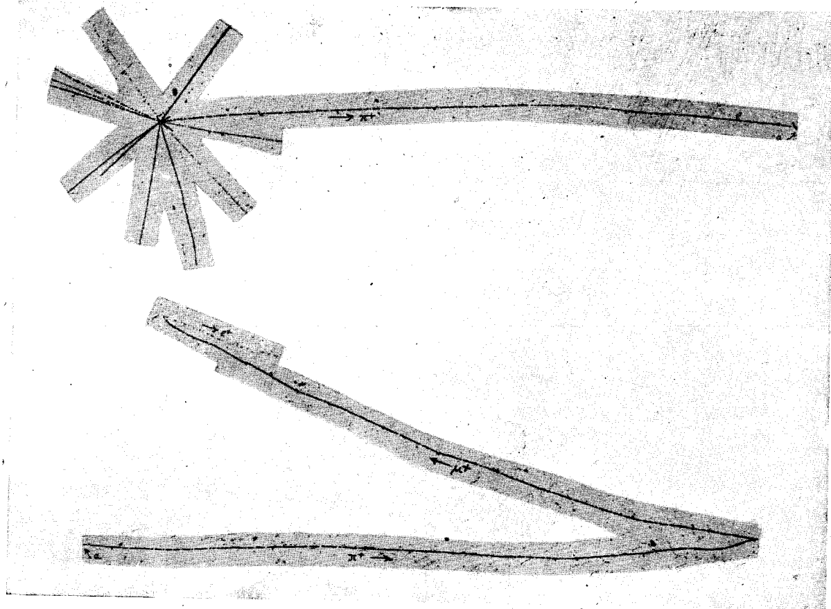
Микрофотография V. Ядерный взрыв, сопровождающийся испусканием \pi^+ -частиц. Показаны две части следа частицы, соединяющиеся в точке a . \pi^+ -частица испытывает последовательный \pi^+ - \mu^+ - e^+ -распад.
