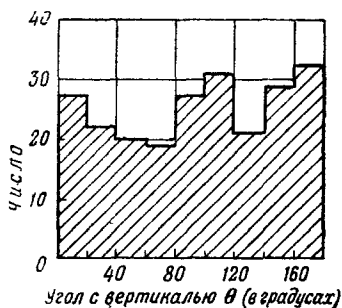
Рис. 16. Распределение направлений испускания \mu^+ -мезонов относительно вертикали, образованных остановившимися в эмульсии \pi^+ -мезонами космического излучения.
