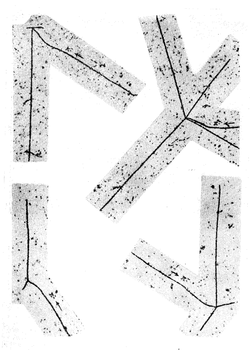
Микрофотография II. Расщепления ядер лёгких элементов, присутствующих в эмульсии (углерод, кислород и азот), при захвате \pi -частиц.
