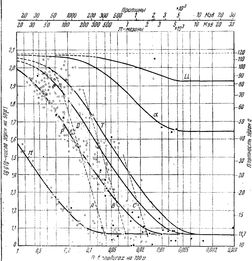
Рис. 10. Распределение значений \alpha (параметр рассеяния) и g (плотность зёрен) для частиц, образованных в звёздах ^{36} . Метод 1.
