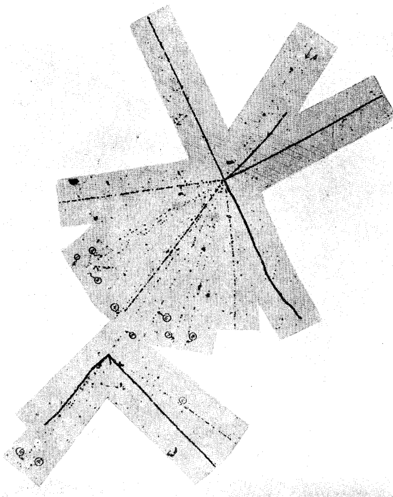
Микрофотография VI. Характерная двойная звезда. Одна из ливневых частиц, созданная в ядерном взрыве, образует вторичное расщепление.
