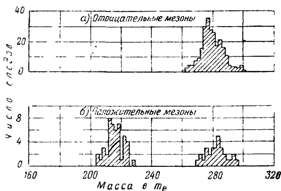
Рис. 6. Распределение значений масс: а) \pi^- и б) \pi^+ и \mu^+ -мезонов, определённых Баркасом и другими методом В.
