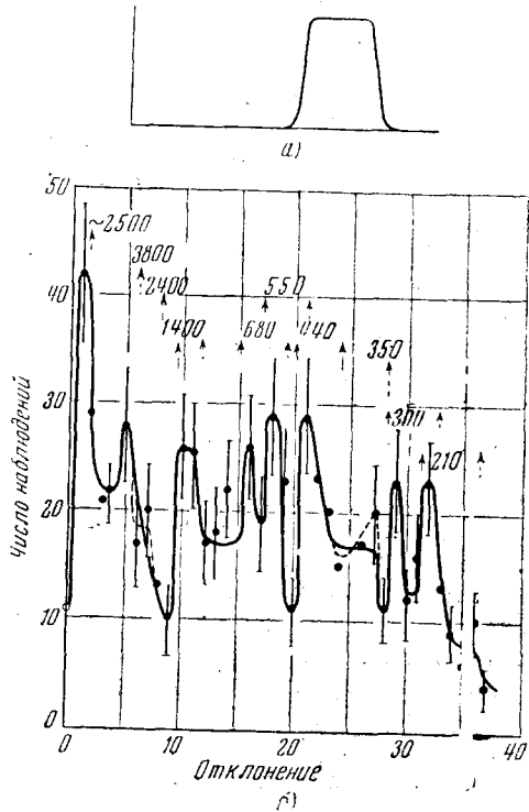
Рис. 40. Типичный результат Алиханяна и др.
