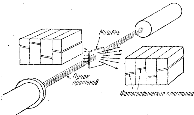
Рис. 22. Аппаратура, использованная для изучения образования мезонов пучком 345- Мэв протонов.
