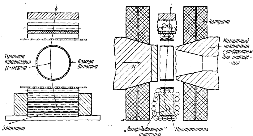
Рис. 18. Установка для определения времени жизни \mu -мезонов 71 . Знак заряда проходящих частиц определяется по значению их отклонения в камере Вильсона, находящейся в магнитном поле.
