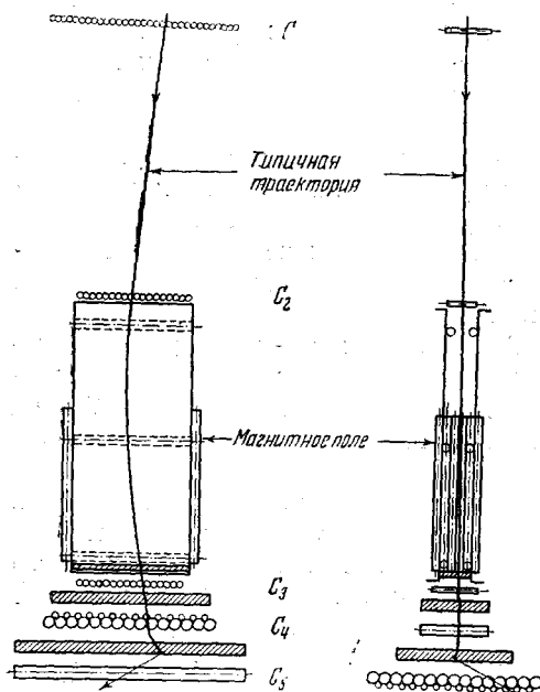
Рис. 39. Установка Алиханяна, Алиханова и Вайсенберга для определения масс заряженных частиц космических лучей.
