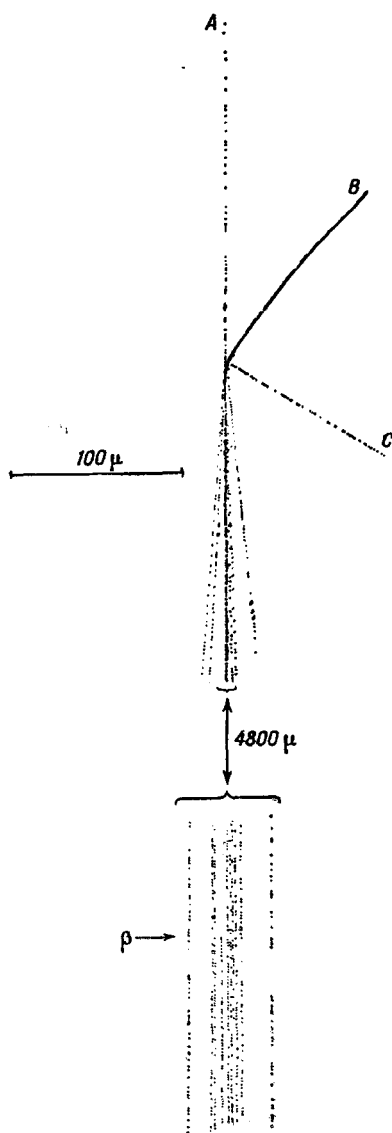
Рис. 1. Микропроекция звезды, образованной протоном сверхвысокой энергии — 3 \cdot 10^{13} эв.
