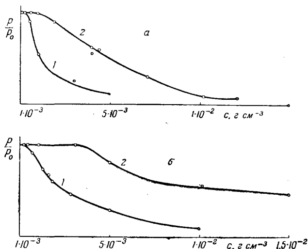
Рис. 8. Концентрационное тушение растворов кислых красителей: a — водного раствора флуоресцеина; б — щелочного раствора натриевой соли перилентетракарбоновой кислоты. 1 — тушение в кювете; 2 — тушение в пористом стекле (по измерениям Ф. М. Пекерман).
