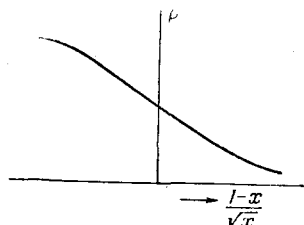
Рис. 1. Вероятность P как функция \frac{1-x}{\sqrt{x}} , где
