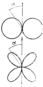
Рис. 5. Плоские диаграммы пространственного излучения электрического диполя и квадруполя.
