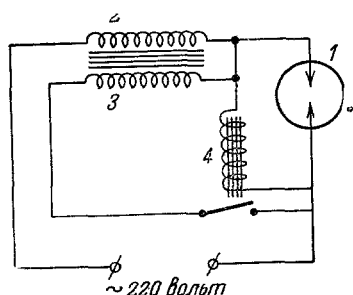
Рис. 11. Принцип конструкции специального дросселя для ртутных ламп СВД, уменьшающего время разгорания.
