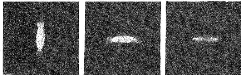
Рис. II. Дуга ртутной лампы сверхвысокого давления, стабилизированной электродами: a — горящей вертикально; б — горящей горизонтально; в — горящей горизонтально, но вращаемой со скоростью 600 об/мин; г , д и е — то же, что a , б и в , но снято через красный фильтр, задерживающий излучение факела дуги.
