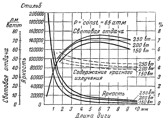
Рис. 7. Зависимость яркости, световой отдачи и содержания красного излучения от длины дуги.
