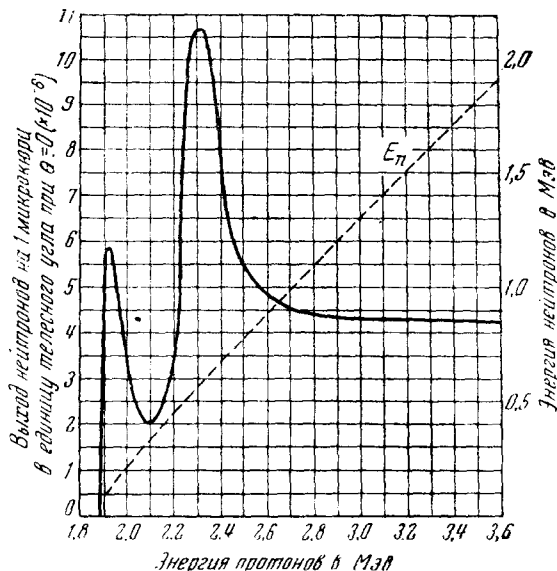
Рис. 23. Выход нейтронов в реакции Li^7(p, n)Be^7 под углом \theta = 0 из мишени толщиной 40 kэв . Пунктирная кривая — энергия нейтронов.
