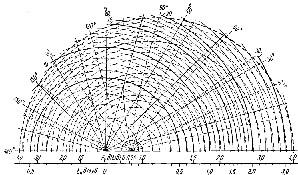
Рис. 32. Номограмма для определения энергии нейтрона в реакции T^3(p, n)He^3 .
