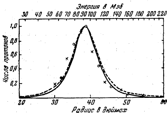
Рис. 19. Спектр протонов при разрыве дейтронов с энергией 190 Мэв. Кривая — вычислена теоретически (по Серберу).
