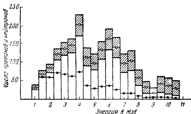
Рис. 5. Спектр нейтронов \text{Ra} + \text{Be} , измеренный по пробегам протонов отдачи в фотоэмульсии. • — протоны, ○ — нейтроны.
