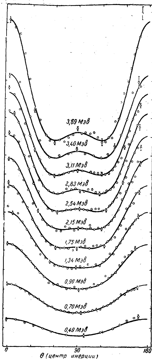
Рис. 9. Угловое распределение нейтронов в реакции D(d, n) He^3 при разных энергиях дейтронов (в координатах центра инерции).
