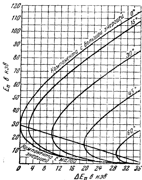
Рис. 28. Энергия нейтронов в реакции \text{Li}^7(p, n)\text{Be}^7 как функция избытка энергии протона над порогом \Delta E_p = E_p - 1,882 для различных углов вылета.
