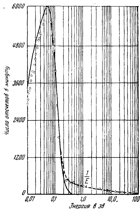
Рис. 36. Спектр нейтронов, выходящих из глубины урано-дейтериевого котла, измеренный при помощи кристаллического спектрометра. Сплошная кривая — распределение Максвелла при T = 400^\circ \text{K} , пунктир — 1/E .
