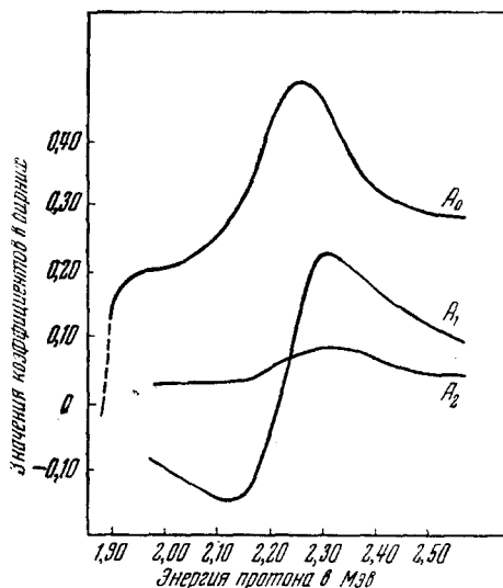
Рис. 26. Коэффициенты разложения углового распределения нейтронов в реакции \text{Li}^7(p, n) в ряд по сферическим функциям в зависимости от энергии протона.
