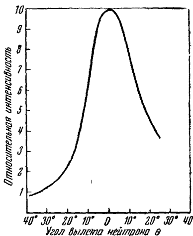
Рис. 13. Угловое распределение нейтронов при бомбардировке \text{LiBO}_2 дейтеронами с энергией 15 Мэв.
