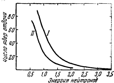
Рис. 35. Спектр нейтронов деления по Цинну и Сцилларду. Кривая I — ядра отдачи He, кривая II — протоны отдачи.
