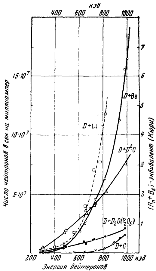
Рис. 7. Выход нейтронов в реакции (d, n) с различными мишенями.
