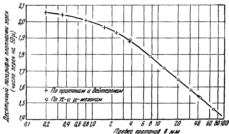
Рис. 24. Плотность зёрен в следе протона как функция её остаточного пробега.
