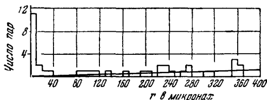
Рис. 48. Наблюдавшееся распределение величин r для r < 400 \mu . Ясно видна группа «коррелированных» пар, наблюдавшаяся при малых величинах r .
