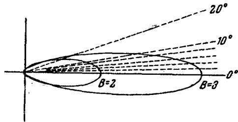
Рис. 52. Полярная диаграмма, показывающая распределение интенсивности \gamma -лучей, образованных при распаде моноэнергетических пучков нейтральных мезонов различных энергий по углам.
