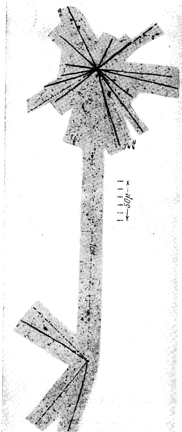
Микрофотография XIII. Наблюдается ливневая частица, испущенная в звезде типа 18+5_p , которая образует вторичное ядерное расщепление типа 5+0_p . Соединяющий след имеет длину 10\,600\ \mu и отождествлен как мезон ( \alpha = 0,049^\circ/100\ \mu ; плотность зёрен равна 10,4 зерна на 50\ \mu ).
