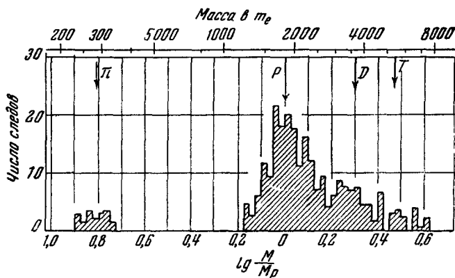
Рис. 27. Распределение масс частиц заряда |e| , соответствующее измерениям, приведённым на рис. 26.
