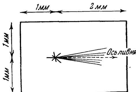
Рис. 47. Площадь вокруг «ливня», которая подробно исследовалась в поисках пар.
