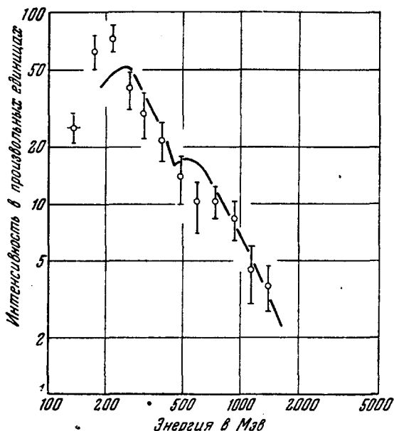
Рис. 33. Дифференциальный спектр полной энергии для мезонов, испускаемых в звёздах. Сплошная кривая — спектр Сандса.
