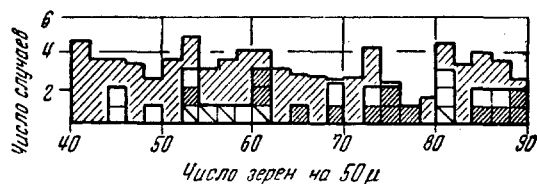
Рис. 35. Распределение по плотности зёрен следов частиц, вызывающих вторичные расщепления. Соответствующее распределение, уменьшенное в 10 раз, для всех следов, выходящих из звёзд, представлено заштрихованной площадью.
