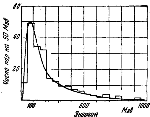
Рис. 38. Распределение энергий пар электронов, наблюдавшихся на высоте 23 км. Гладкая линия показывает ожидаемый спектр фотонов, возникающих при распаде нейтральных мезонов с массой 280 m_e и кинетической энергией заряженных \pi -мезонов, образованных в «звездах».
