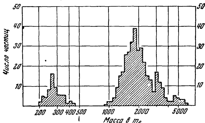
Рис. 30. Распределение масс частиц с зарядом |e| , соответствующее результатам, представленным на рис. 29.
