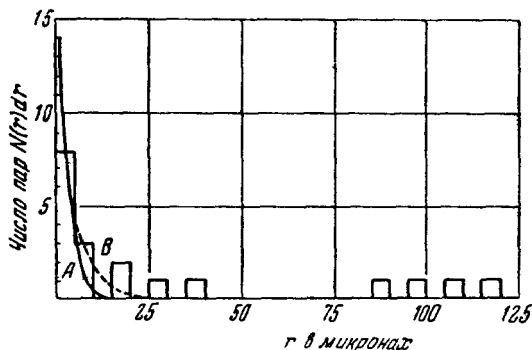
Рис. 50. Распределение наблюдавшихся величин r для коррелированных пар. Кривые A и B изображают ожидаемые распределения величин r , обусловленные вероятными ошибками 0,25 и 0,5^\circ измерений направления движения фотона. Время жизни мезона предположено бесконечно малым.
