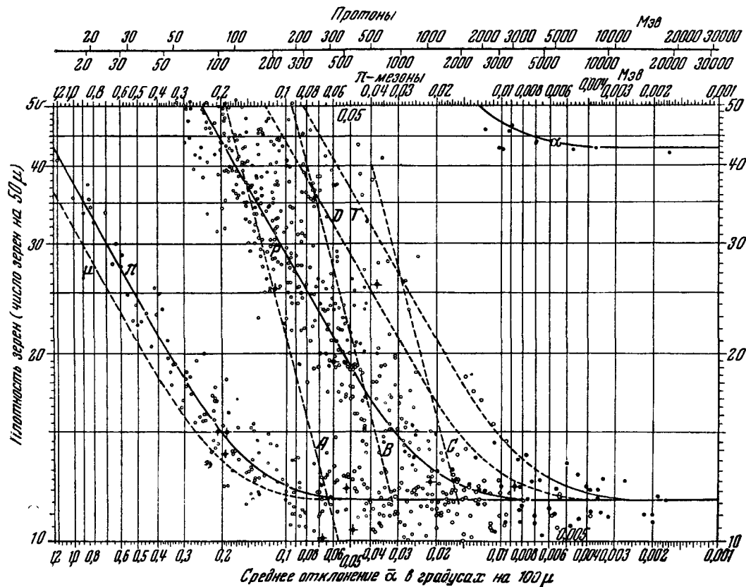
Рис. 29. Зависимость плотности зёрен от \bar{\alpha}^\circ (100 μ) для следов 700 частиц. ● — первичные частицы, ○ — вторичные частицы, ○ — частицы, соединяющие двойные звёзды. Кривые \mu , \pi , \rho , D , T означают то же, что на рис. 26. A , B , C — ливни, соответствующие постоянному импульсу, равному соответственно 500, 1000 и 2000 Мэв/с. Кинетическая энергия протонов и \pi -мезонов дана в верхней части рисунка.
