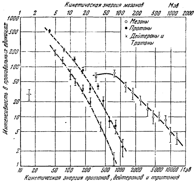
Рис. 32. Дифференциальный спектр кинетической энергии для частиц различных типов. Точка, соответствующая энергии мезонов 1,6 Мэв, получена только для \pi^- -мезонов, образованных в звёздах и создающих на конце пробега ядерное расщепление. Для получения числа частиц на звезду на интервал энергии в 1 Мэв надо умножить соответствующие значения приблизительно на 2,5 \cdot 10^{-5} .
