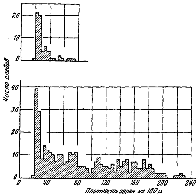
Рис. 28. Распределение величин плотности зёрен в следах частиц с зарядом |e| . На нижнем рисунке — распределение для всех частиц, на верхнем — для частиц, идентифицированных как \pi -мезоны.
