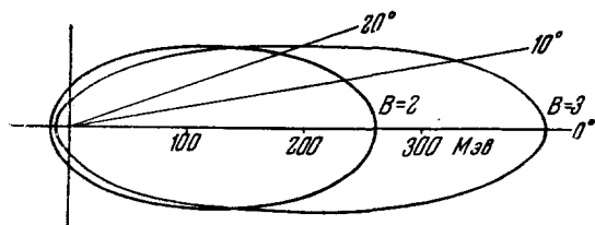
Рис. 41. Полярная диаграмма, показывающая зависимость энергии фотонов от направления их испускания, если фотоны образовались при распаде нейтральных мезонов. Вычисления проделаны для двух величин полной энергии нейтральных мезонов.
