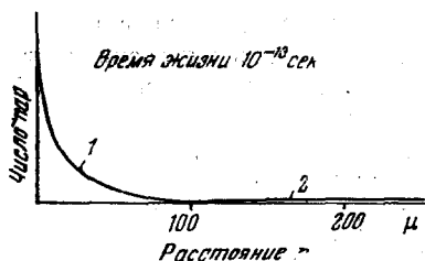
Рис. 46. 1 — вычисленное распределение величин r для предположенного времени жизни нейтрального мезона 10^{-13} сек.; 2 — вычисленное распределение, обусловленное случайными парами.
