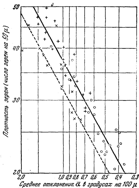
Рис. 31. Зависимость между плотностью зёрен и \bar{\alpha}^\circ (100 \mu ). о — мезоны, испущенные из звёзд, те же самые, что и на рис. 29 для соответствующего интервала плотности зёрен; + — \pi -мезоны, либо распадающиеся на \mu -мезон, либо дающие звезду на конце пробега; x — \mu -мезоны, распадающиеся на конце пробега на электрон.
