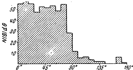
Рис. 39. Угловое распределение направлений движения фотонов на высоте 23 км.
