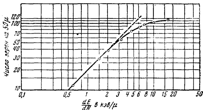
Рис. 25. Соотношение между плотностью зёрен и удельной потерей энергии вдоль следа. Эмульсия Ильфорд G-5.
