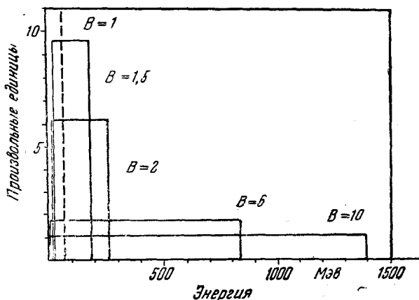
Рис. 42. Распределение энергий фотонов, образованных при распаде моноэнергетических нейтральных мезонов.
