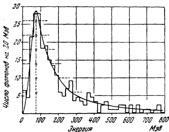
Рис. 43. Спектр \gamma -излучения на высоте 23 км. Гладкая линия — это линия, дающая наилучшее согласие с экспериментальными результатами; масса нейтрального мезона вычислена из неё.
