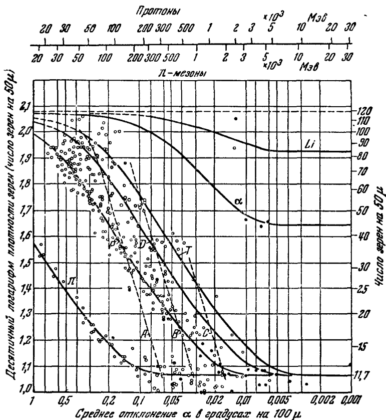
Рис. 26. Соотношение между плотностью зёрен и \alpha (100 м) для следов 350 частиц. «Первичные» частицы обозначены \bullet , «вторичные» частицы — \circ . Кривая P имеет такую же форму, как и вычисленная кривая для протонов, но она смещена влево вдоль \alpha -оси на 7%. Линии \pi , D и T проведены в правильном соотношении с линией P , чтобы соответствовать частицам с массой 286 m_e , 3674 m_e и 5511 m_e . A , B и C являются линиями постоянного импульса и соответствуют импульсам 500, 1000 и 2000 Мэв/с. Шкалы энергии (в Мэв) для \pi -мезонов и протонов приведены в верхней части рисунка. Видно, что все \alpha -частицы большой энергии являются «первичными» частицами. Две точки, соответствующие частицам большей массы, принадлежат «первичному» ядру азота и «вторичному» ядру лития, возникшему в том же самом акте.
