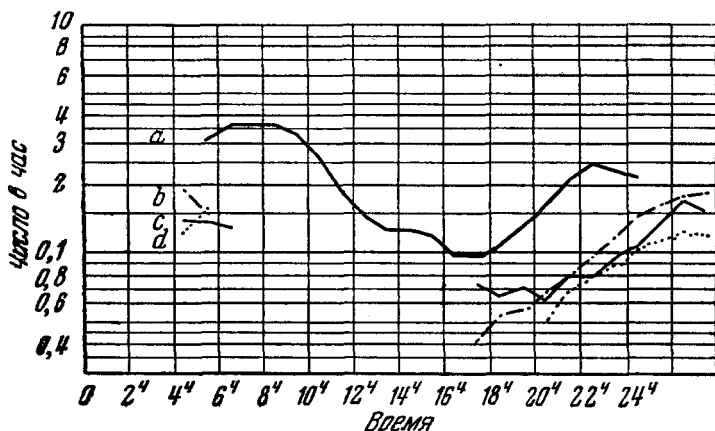
Рис. 11. Суточная вариация численности «вспышек» и метеоров. a —среднее число вспышек в час; февраль 1943—январь 1944 гг., b —число метеоров в час по наблюдениям Шмидта, c —то же по наблюдениям Кувье-Гравье, d —то же по наблюдениям Гофмейстера.
