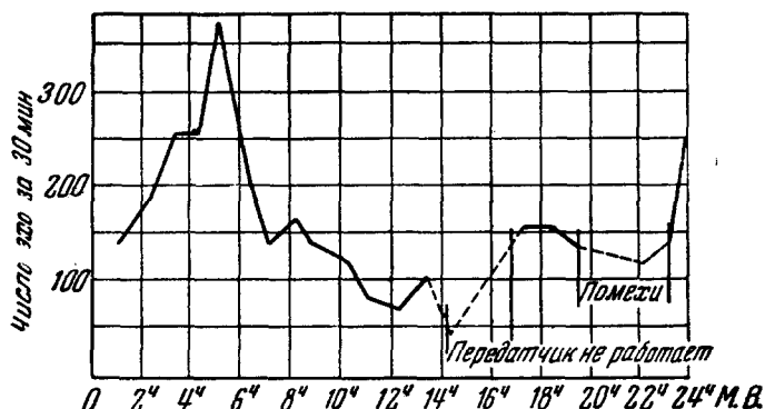
Рис. 9. Счёт числа эхо на волне 39,5 м при наблюдениях 15—16 октября 1938 г.
