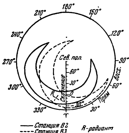
Рис. 18. Области возможных положений радианта, соответствующие главным максимумам часовых чисел для станций В2 и В3.
