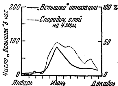
Рис. 6. Годичные вариации численности «вспышек» ионизации и частоты появления спорадического слоя E в дневное время (среднее за 1944—1946 гг.).
