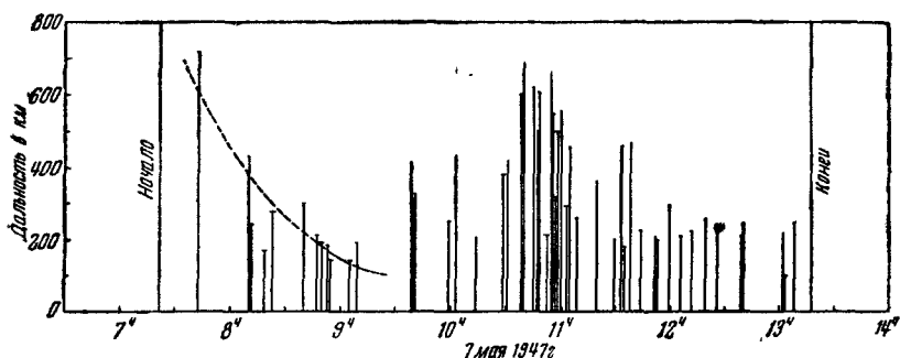
Рис. 19. Дальности эхо в функции времени. Наблюдения 7 мая 1947 г. с узким лепестком излучения, направленным на восток с целью определения положения радиантов по методу Клегга. Между 7 ч 30 м и 9 ч 30 м наблюдалось прохождение через луч радианта Эта-акварид (пунктиром показана теоретическая кривая дальностей). Дальнейшие эхо принадлежат новому дневному потоку, прохождение которого начинается в 10 ч 35 м (поток из созвездия Рыб).
