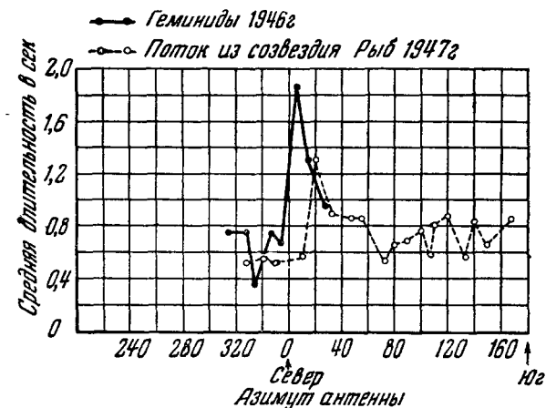
Рис. 24. Средние длительности эхо в зависимости от направления наблюдений.
