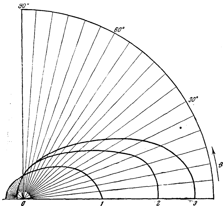
Рис. 12. Кривая 1 — электрический диполь l=1 , кривая 2 — электрический октополь l=3 , кривая 3 — магнитный квадруполь l=2 . k=5 . Импульс электрона \mathbf{r} направлен по лучу \vartheta=0 . Вероятность образования пары при \vartheta=90^\circ для всех трёх кривых принята равной 1.
