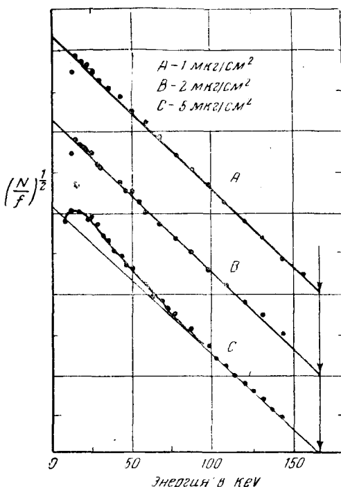
Рис. 6. График Ферми для \beta -спектра \text{S}^{35} .
