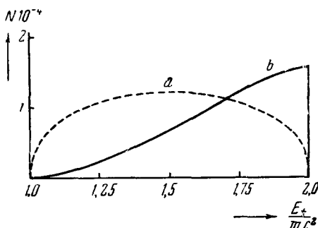
Рис. 13. a — борновское приближение ( l=2 ), b — Z=84 ( l=2 ).
