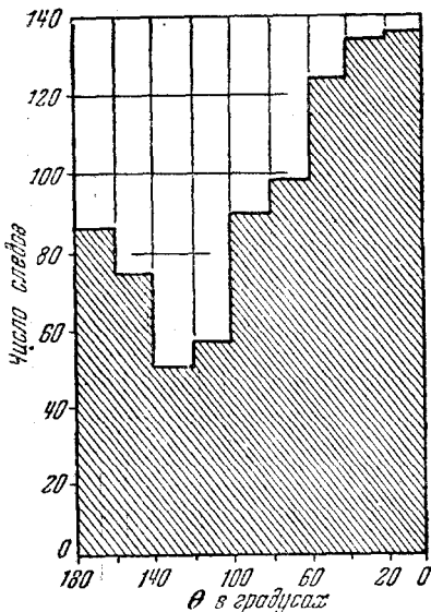
Рис. 18. Распределение величин \theta для всех тонких следов, связанных со звёздами, наблюдавшихся на серии пластинок, экспонированных на большой высоте. \theta — угол между вертикалью и проекцией следа на плоскость эмульсии.
