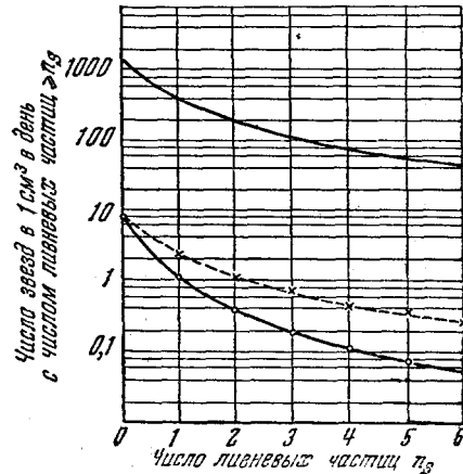
Рис. 19. Частота образования звёзд с различным числом n_s на высотах 21 200 м и 3300 м. Для сравнения приведена пунктирная кривая, иллюстрирующая результаты, относящиеся к высоте 21 200 м и нормированные так, чтобы полные частоты образования звёзд на высоте 21 200 м и 3300 м были равны.
