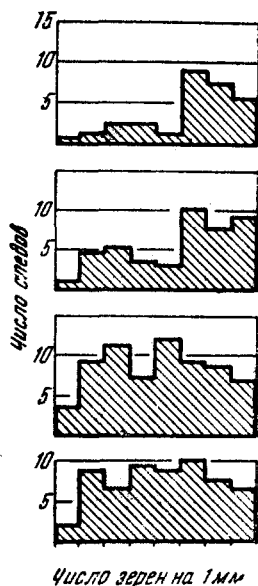
Рис. 14. Диаграмма, показывающая распределение плотности зёрен «серых» следов, связанных со «звёздами» различных классов.
