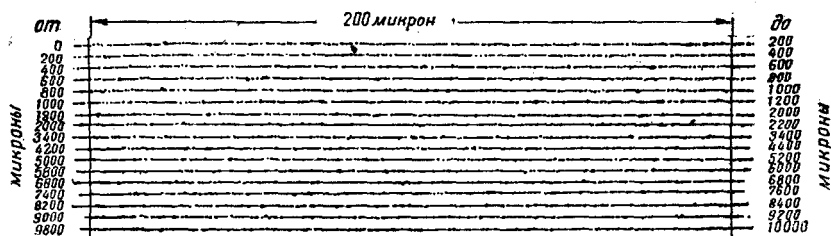
Рис. 21. Изображение последовательных элементов (каждый из которых длиной 200 \mu ) следа ливневой частицы с полной длиной 10 000 \mu . След прямолинеен с точностью 0,03°, а энергия частицы, которая его образует, должна быть больше чем 1,5 \cdot 10^9 эв.
