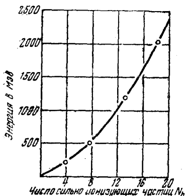
Рис. 2. Средняя энергия, освобожденная в «звездах», в которых образовано различное число сильно ионизирующих частиц. Величины энергии соответствуют энергии испущенных нуклонов и не включают энергию «ливневых» частиц.
