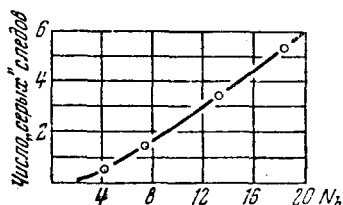
Рис. 15. Среднее число «серых» следов как функция полного числа сильно ионизующих частиц N_h в «звезде».
