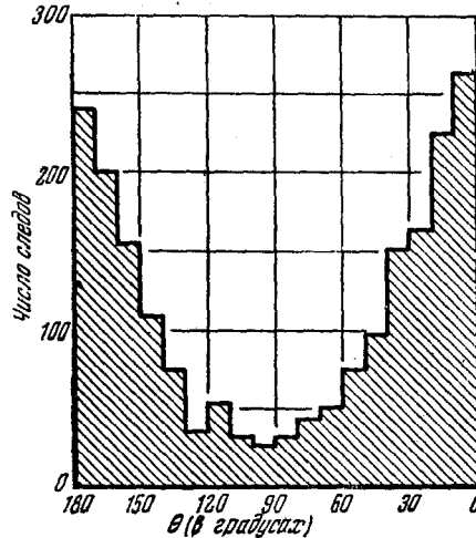
Рис. 4. Распределение величин \theta для следов всех быстрых частиц, связанных со «звёздами». \theta — угол между вертикалью и проекцией следа на плоскость эмульсии. 0^\circ соответствует направлению вертикали, опущенной вниз из центра звезды.
