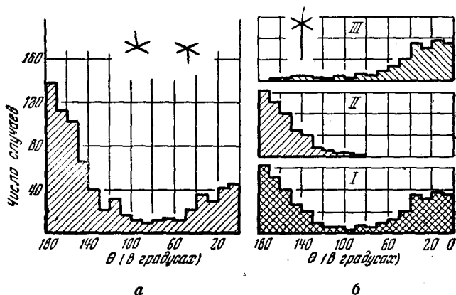
Рис. 5. Распределение величин \theta для следов быстрых частиц; а — для звёзд с одной быстрой частицей; б — для звёзд с двумя быстрыми частицами. На рис. 5, б первоначальные наблюдения (I) были проанализированы, чтобы показать распределение величин \theta для падающих частиц (II) и для вылетающих частиц (III).
