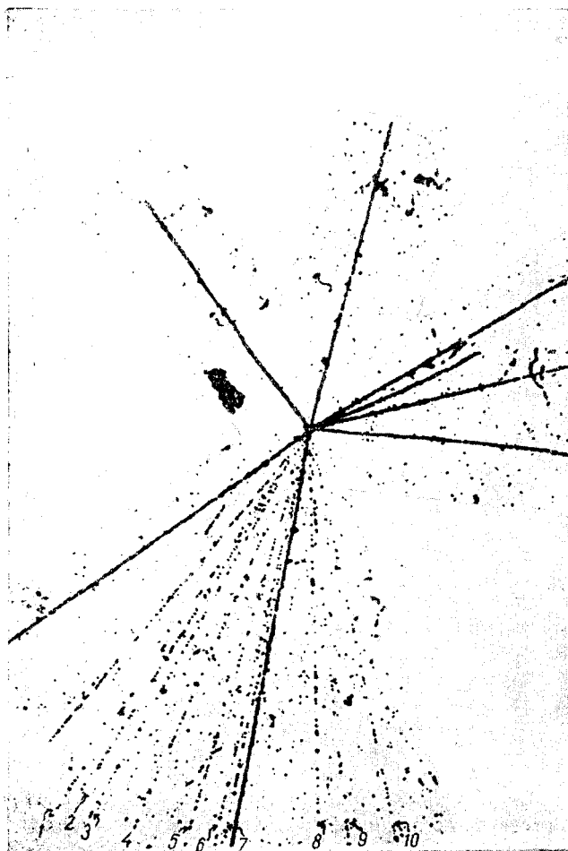
Микрофотография VII. Мозаика «ливня» типа 10_n ( N_h=9 ).
