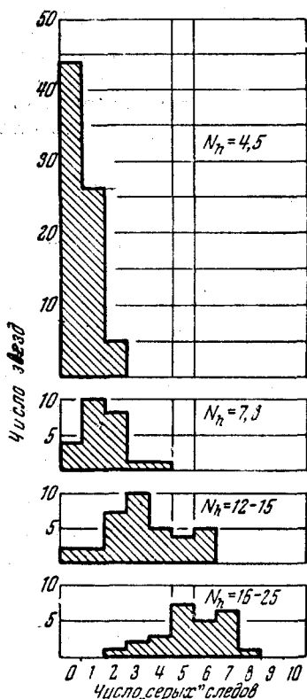
Рис. 13. Диаграмма, показывающая распределение числа «серых» следов в звёздах различных классов.
