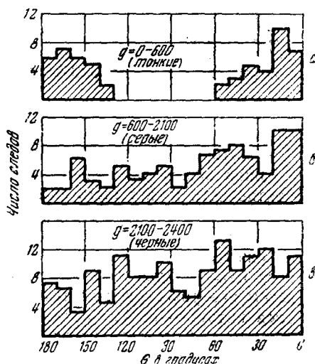
Рис. 3. Распределение величин \theta для «тонких», «серых» и «чёрных» следов. В этом случае наблюдения ограничивались следами, длина которых была больше 300 \mu , связанными со звёздами с семью или большим числом лучей ( N_h \geq 7 ).
