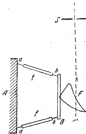
Рис. 4. Схема конструкции призмы для перемещения призмы в монохроматоре Бэкмана. F — призма Фери, B — несущая её площадка, ff — стержни, A — основание, или стенка прибора.
