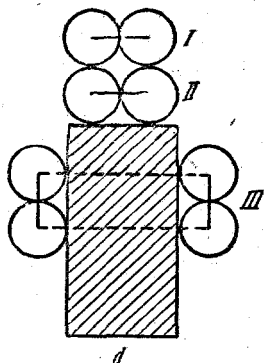
Рис. 22. Схема установки, на которой была подтверждена малая вероятность захвата оставшихся мезонов в лёгких веществах 89 . Счётчики группы III регистрировали электроны от распада мезонов обоого знака в фильтре d .
