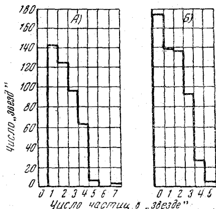
Рис. 31. Распределение ядерных расщеплений, вызываемых «космическими» (А) и «искусственными» (Б) остановившимися мезонами по числу испускаемых заряженных частиц 112 .
