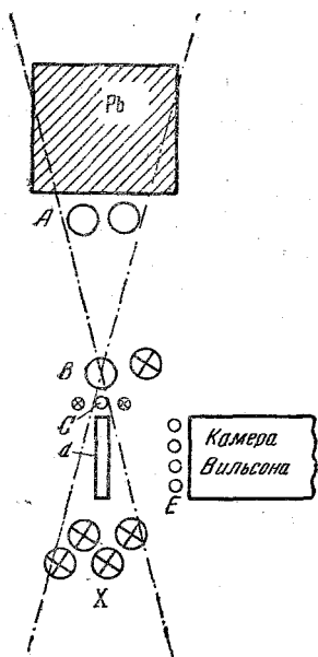
Рис. 17. Схема установки с камерой Вильсона, в которой исследовались энергии электронов от распада мезонов в графитовой пластинке d 68 . Камера Вильсона управлялась от антисовпадений (А, В, С, Е, —Х).
