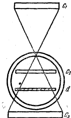
Рис. 13. Схема камеры Вильсона, применявшейся для исследования спектра электронов распада 65 . Камера управлялась антисовпадениями ( C_1 , C_2 , -C_3 ); d — пластинка ( 2 \text{ г/см}^2 графита), предназначенная для поглощения мезонов.
