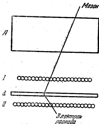
Рис. 2. Схема первой из установок 38 , применявшихся для обнаружения распада остановившихся мезонов.
