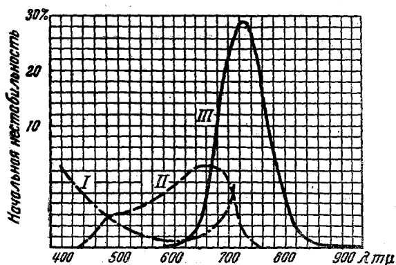
Рис. 9. Изменение начальной неустойчивости по спектру: I — рост тока (Вестон); II — спад тока (Тунгсрам); III — спад тока (САФ.)
