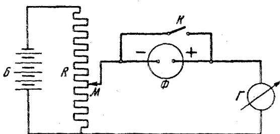
Рис. 17. Схема Вуда: \Phi — фотоэлемент, \Gamma — гальванометр, R — делитель напряжения, М — скользящий контакт, К — ключ, Б — батарея.
