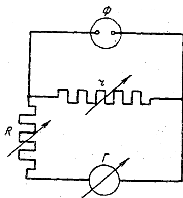
Рис. 19. \Phi — фотоэлемент, G — гальванометр.
