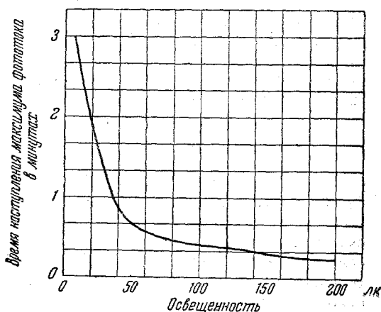
Рис. 8. Время наступления максимума фототока в зависимости от освещённости ( T_{\text{пв}} = 2360^\circ \text{ К} ).
