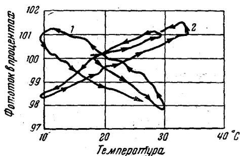
Рис. 13. Влияние внешнего сопротивления на зависимость тока от температуры: I — освещённость 400 лк, R_{вн}=1000 \text{ Ом} ; II — освещённость 400 лк, R_{вн}=0 .
