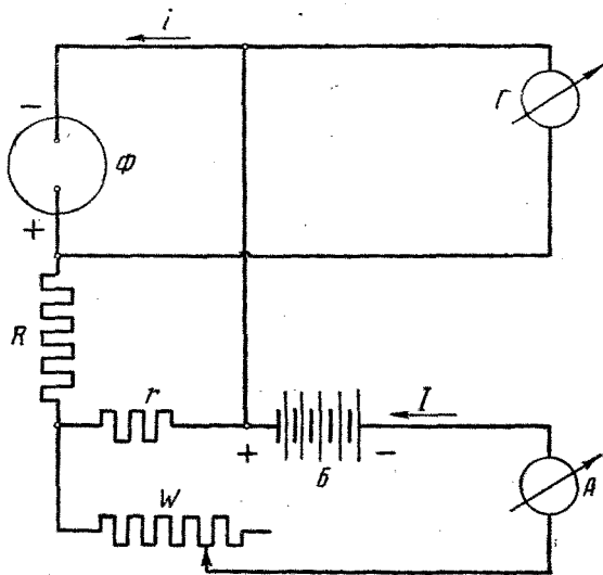
Рис. 18. Схема Фроммера: \Phi — фотоэлемент, \Gamma — гальванометр, А — миллиамперметр, W — реостат, R, r — постоянные сопротивления, Б — батарея.
