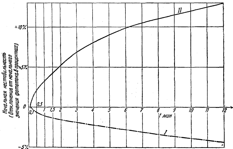
Рис. 6. Начальная неустойчивость: I—ГОИ № 1896 1947 г.; II—ГОИ № 1900 1947 г.
